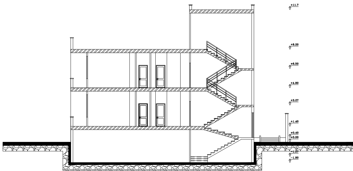
SECTION A.A SC: 1/100
