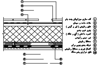
جزئیات عایق حرارتی بام
