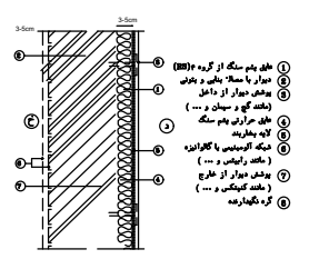
جزئیات عایق حرارتی دیوار خارجی
