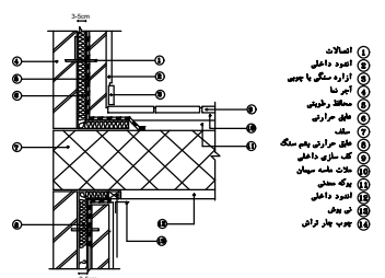
جزئیات عایق حرارتی دیوار جانبی
