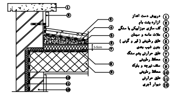
جزئیات عایق حرارتی گوشه بام به دیوار جانبی
