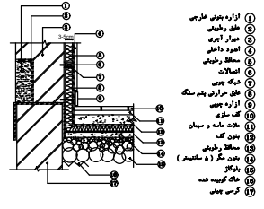
جزئیات عایق حرارتی کف
