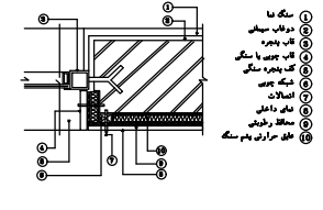
جزئیات عایق حرارتی دیوار به پنجره
