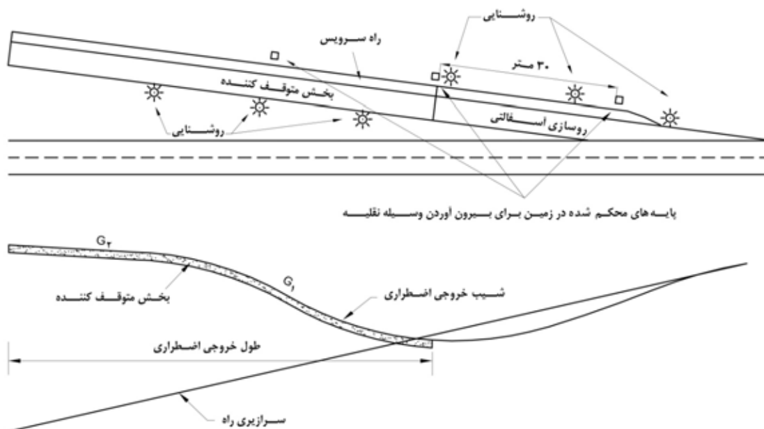
شکل ۵-۲۱- نمونه پلان و نیم‌رخ طولی یک خروجی اضطراری
