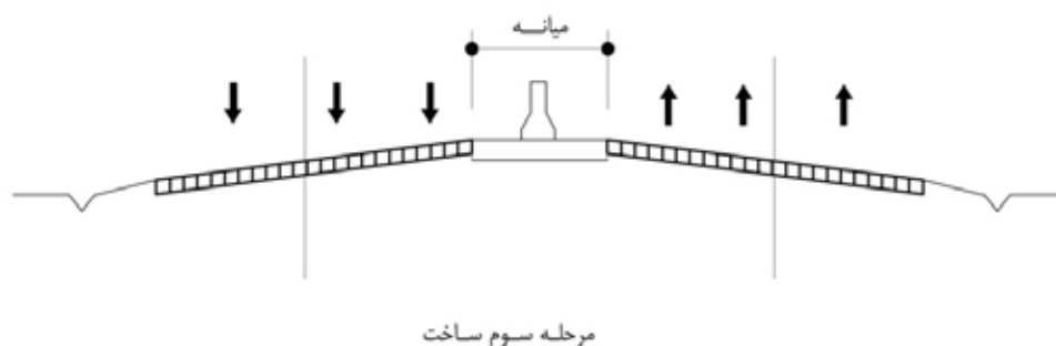
شکل ۴-۹- مرحله سوم ساخت یک راه چند خطه جداشده با میانه کم عرض
