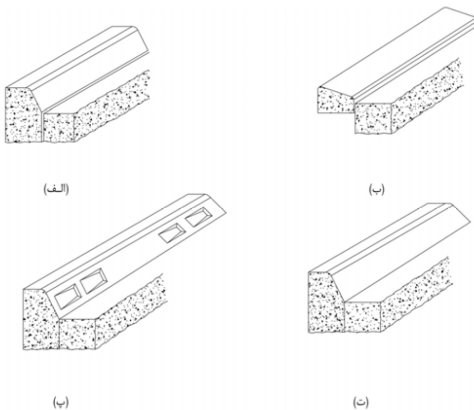
شکل ۶-۲۴- انواع جدول با قابلیت رویت زیاد
