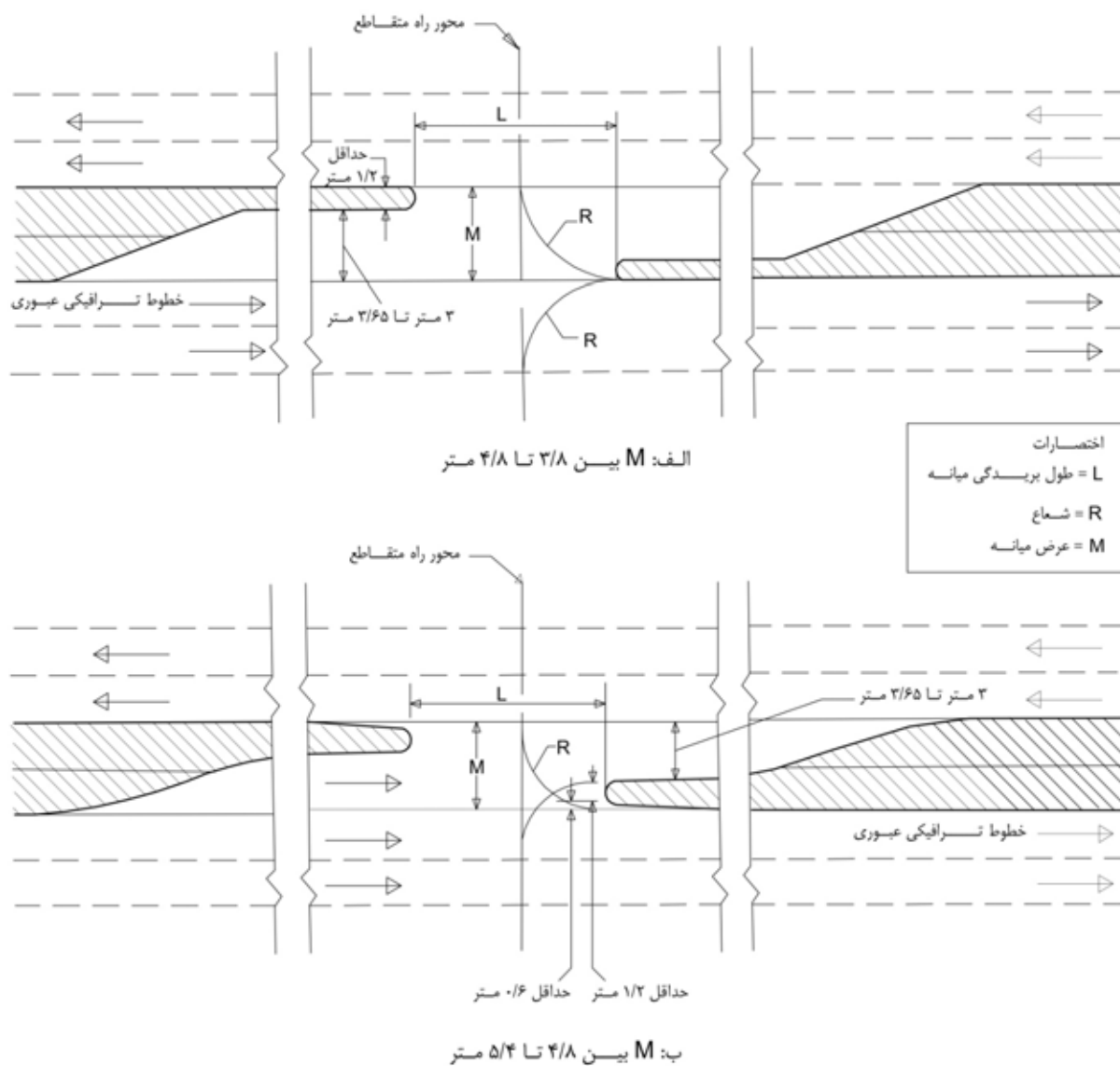
شکل ۸-۴۴- طرح گردش به چپ با خط کمکی در راه‌های دارای میانه ۳/۸ تا ۵/۴ متر
