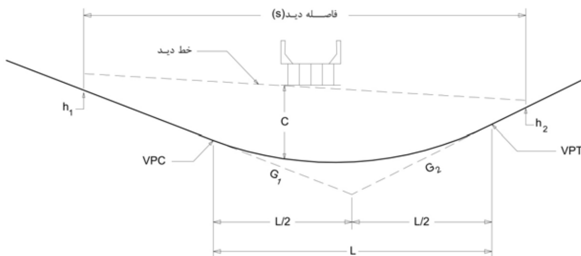
شکل ۵-۱۶- خط دید در خم کاسه‌ای
