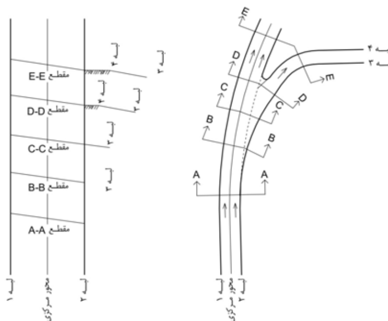
شکل ۸-۳۰- نحوه تأمین بریلندی در پایانه- جداشدگی از قوس هم‌جهت
