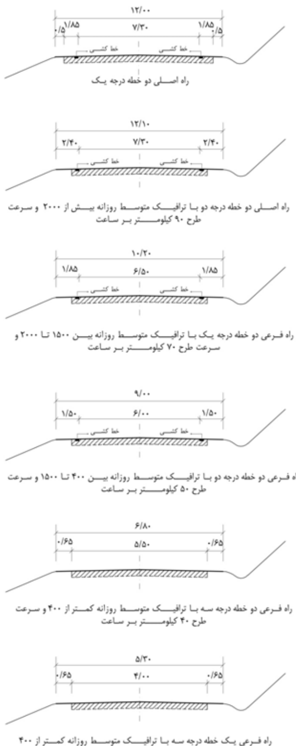
شکل ۶-۲۶- نیمرخ‌های عرضی نمونه برای راه‌های اصلی دو خطه و راه‌های فرعی
