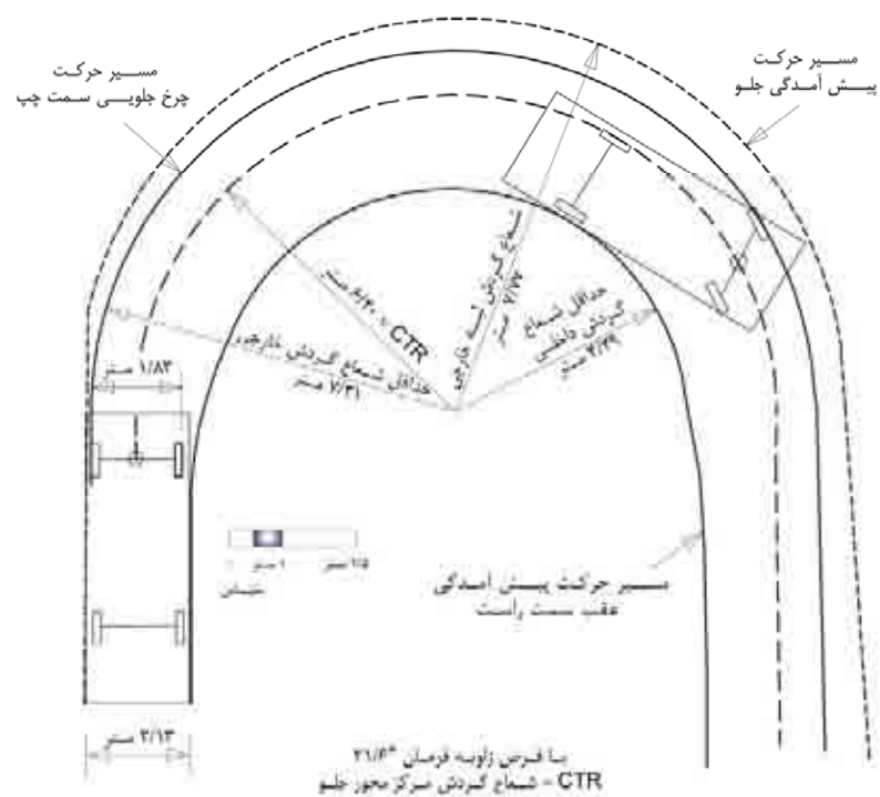
شکل ۴-۱- مشخصات مسیر گردش خودروی طرح، سبک (سواری)
