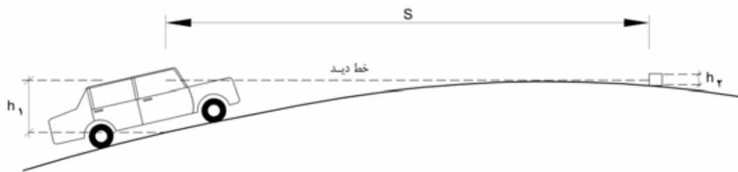
شکل ۵-۱۴ - محدودیت دید در قوس قائم گنبدی
