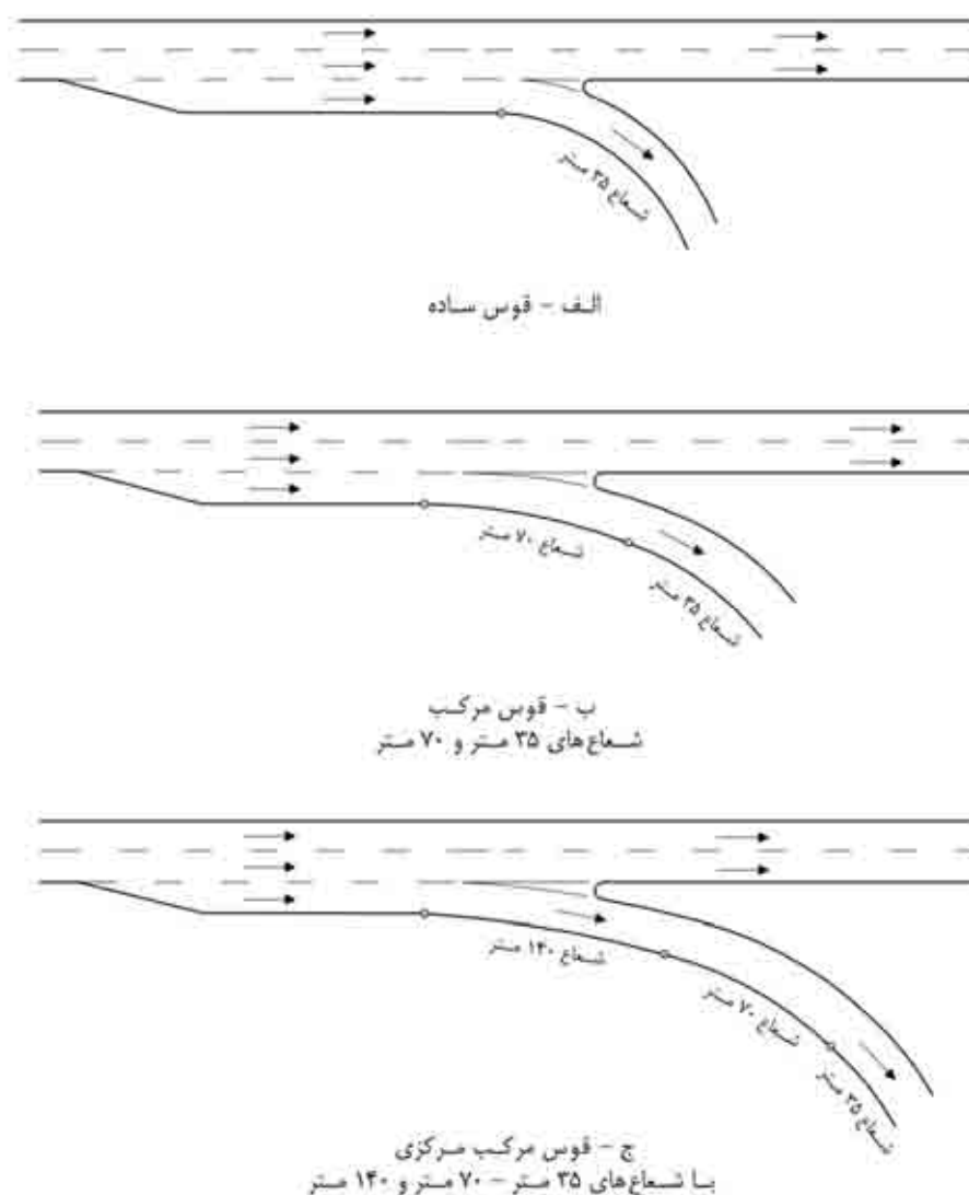
شکل ۸-۲۸- طرح نمونه برای مسیرهای گردش با جریان آزاد
