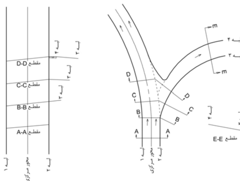
شکل ۸-۳۱- نحوه تأمین بریلندی در پایانه- جداشدگی با قوس غیر هم‌جهت
