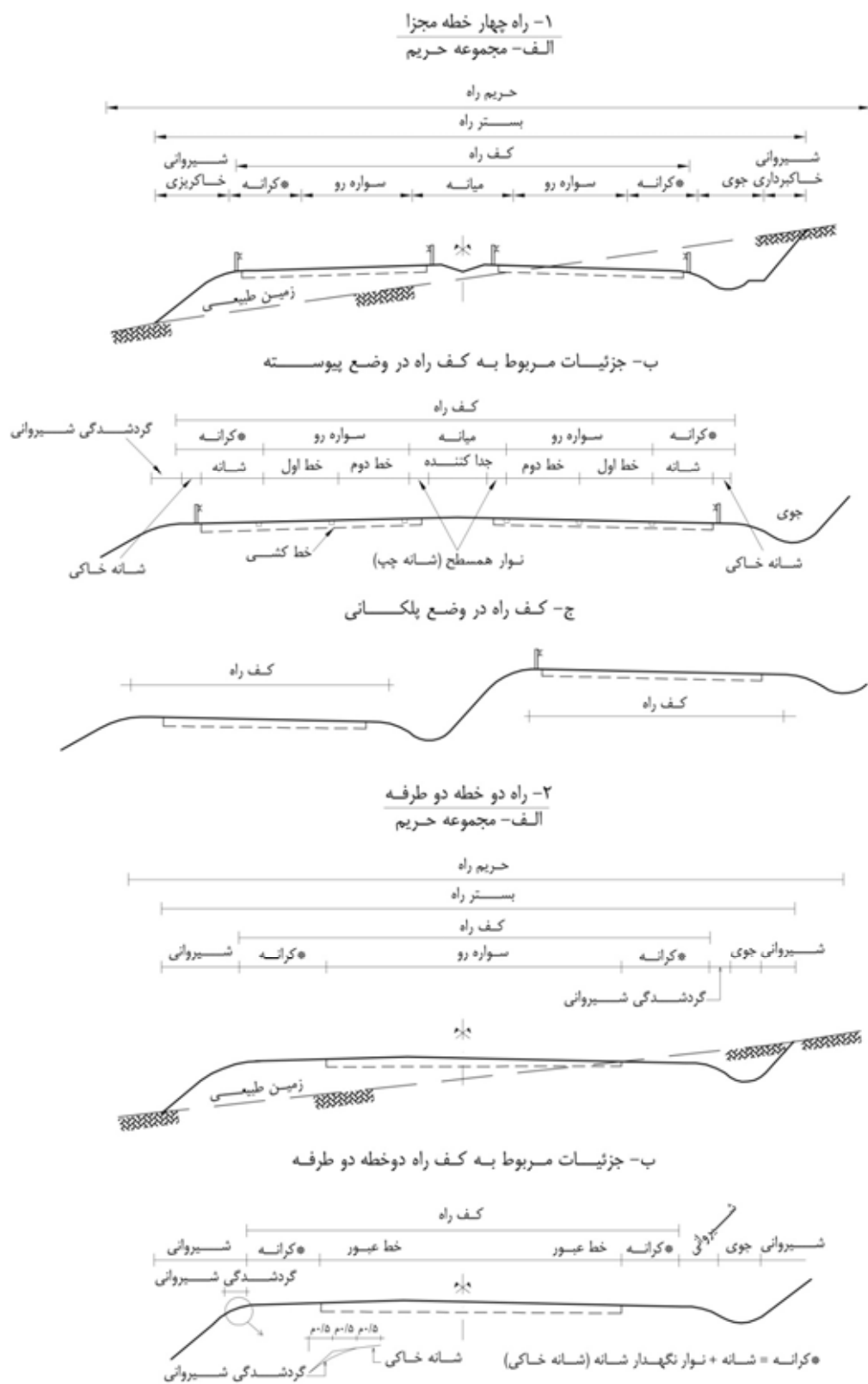
شکل ۲-۶- اجزای نیمرخ عرضی در راه‌های دو خطه و چهار خطه
