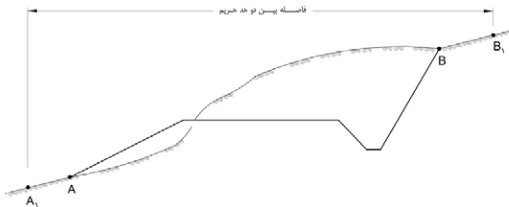
شکل ۵-۶- حریم راه
