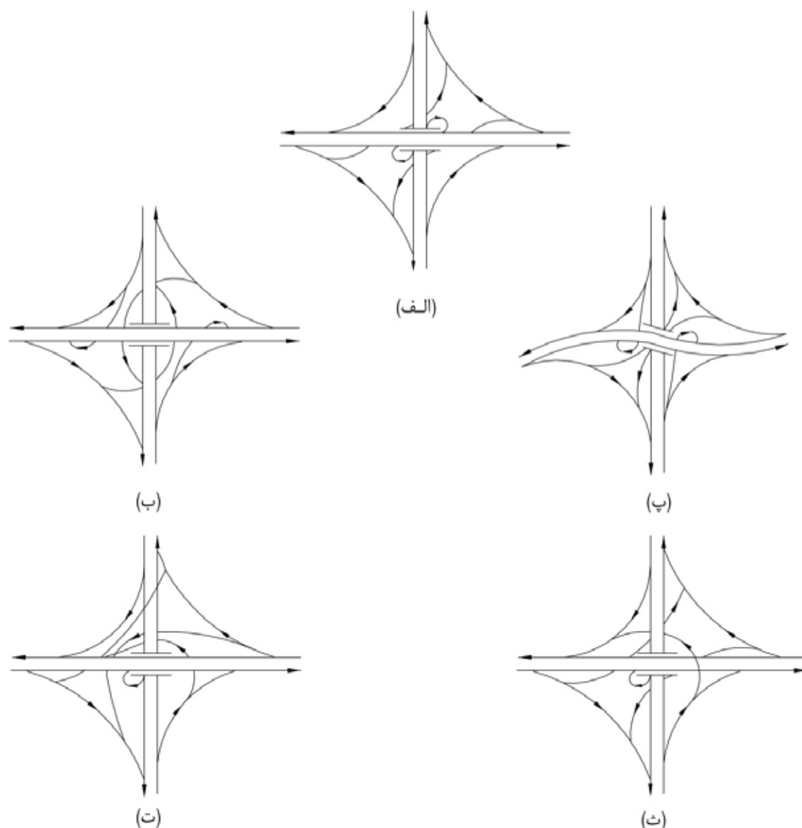
شکل ۹-۱۲- نمونه تبادله‌های نیمه‌جهتی بدون ترافیک تداخلی
