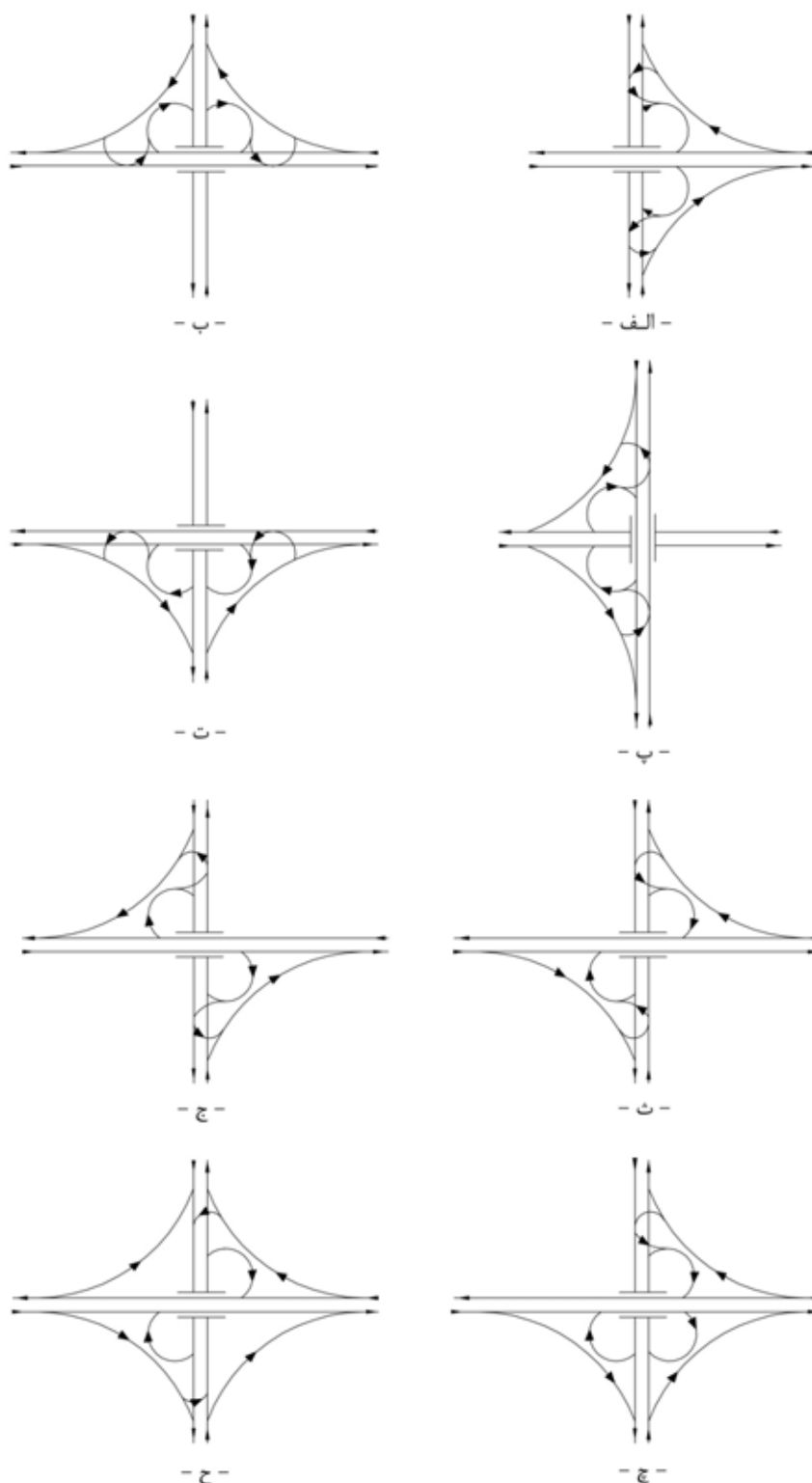
شکل ۹-۹- نمونه طرح‌های ورودی و خروجی تبادلهای نیمه‌شیدری
