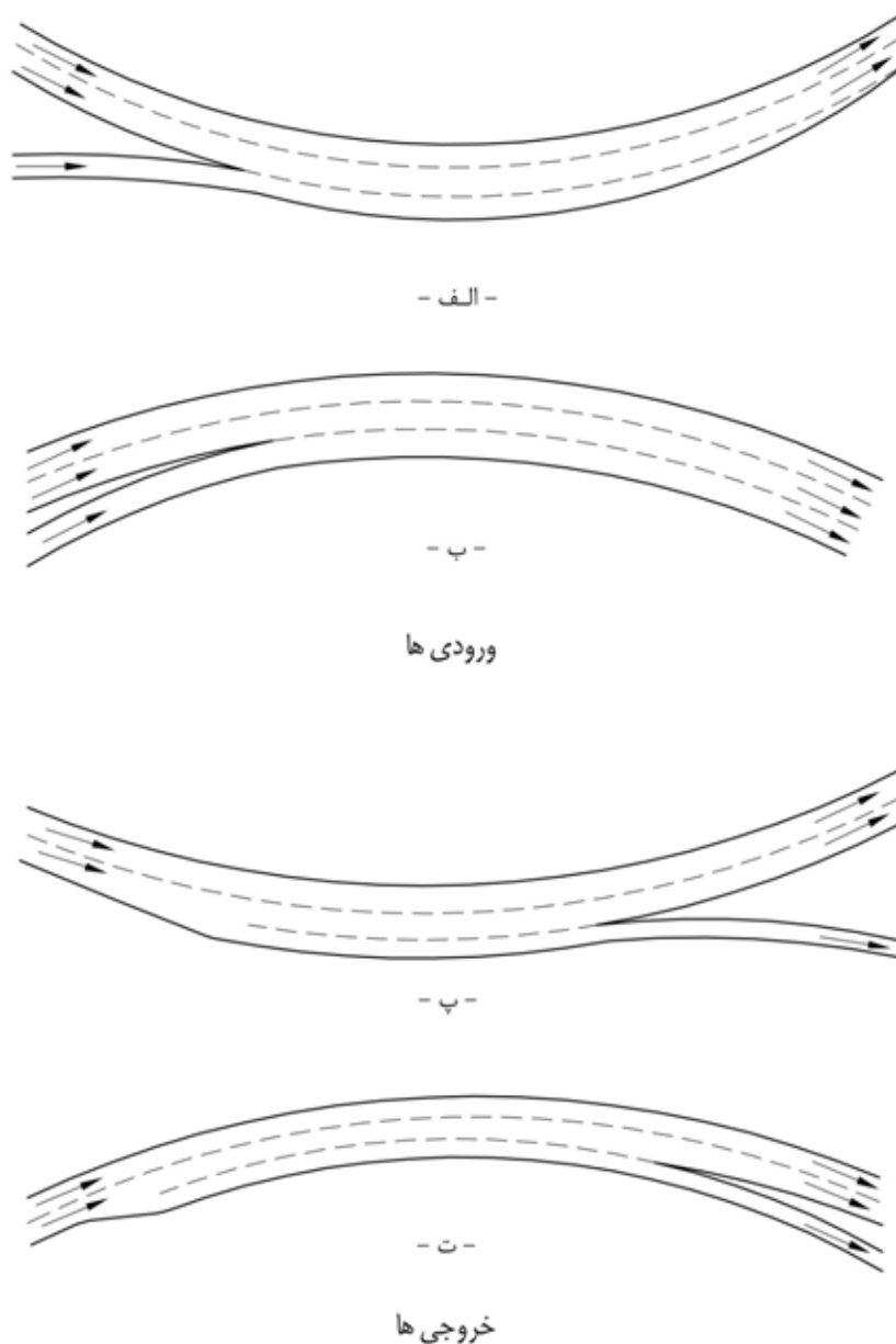
شکل ۹- ۲۶ - حالت شماتیک پایانه‌های رابط نوع موازی واقع در قوس افقی
