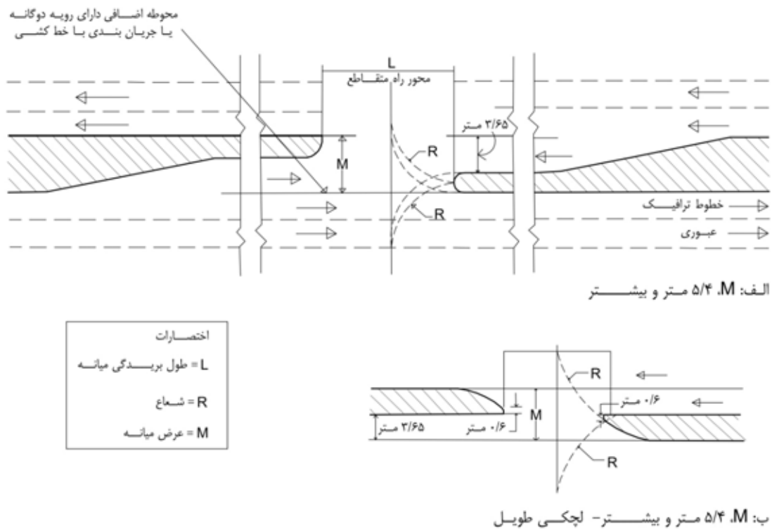
شکل ۸-۴۵- طرح گردش به چپ با خط کمکی در راه‌های دارای میانه بیشتر از ۵/۴ متر
