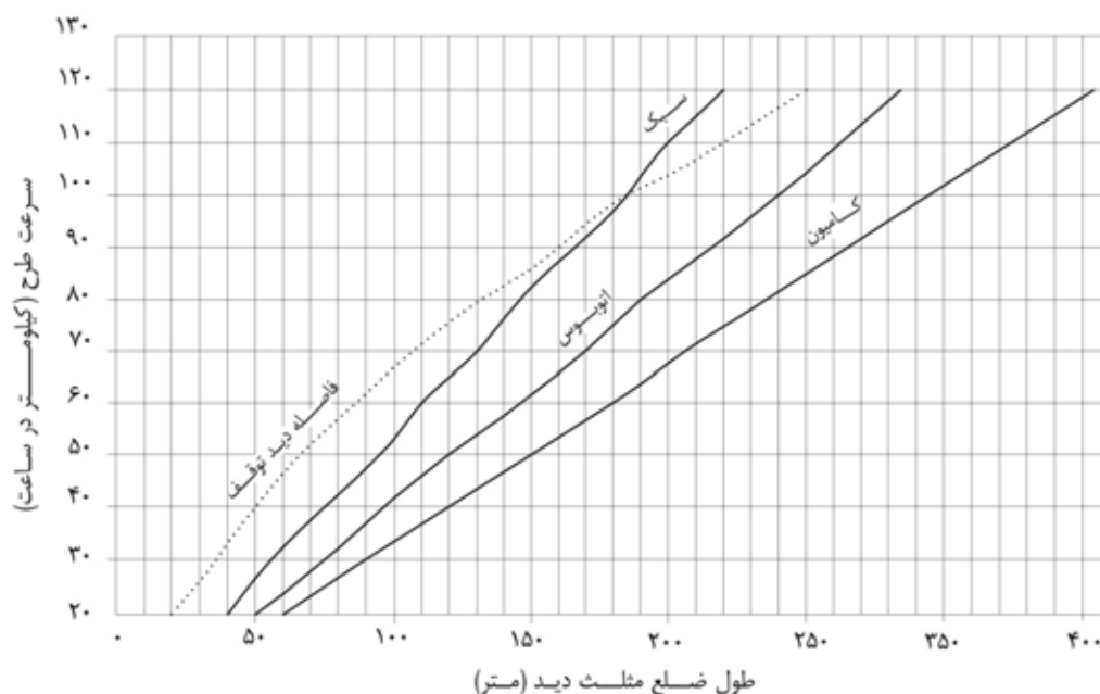
شکل ۸-۳۵- نمودار تعیین فاصله دید تقاطع برای گردش به راست و عبور مستقیم از مسیر فرعی در تقاطع با تابلوی ایست
