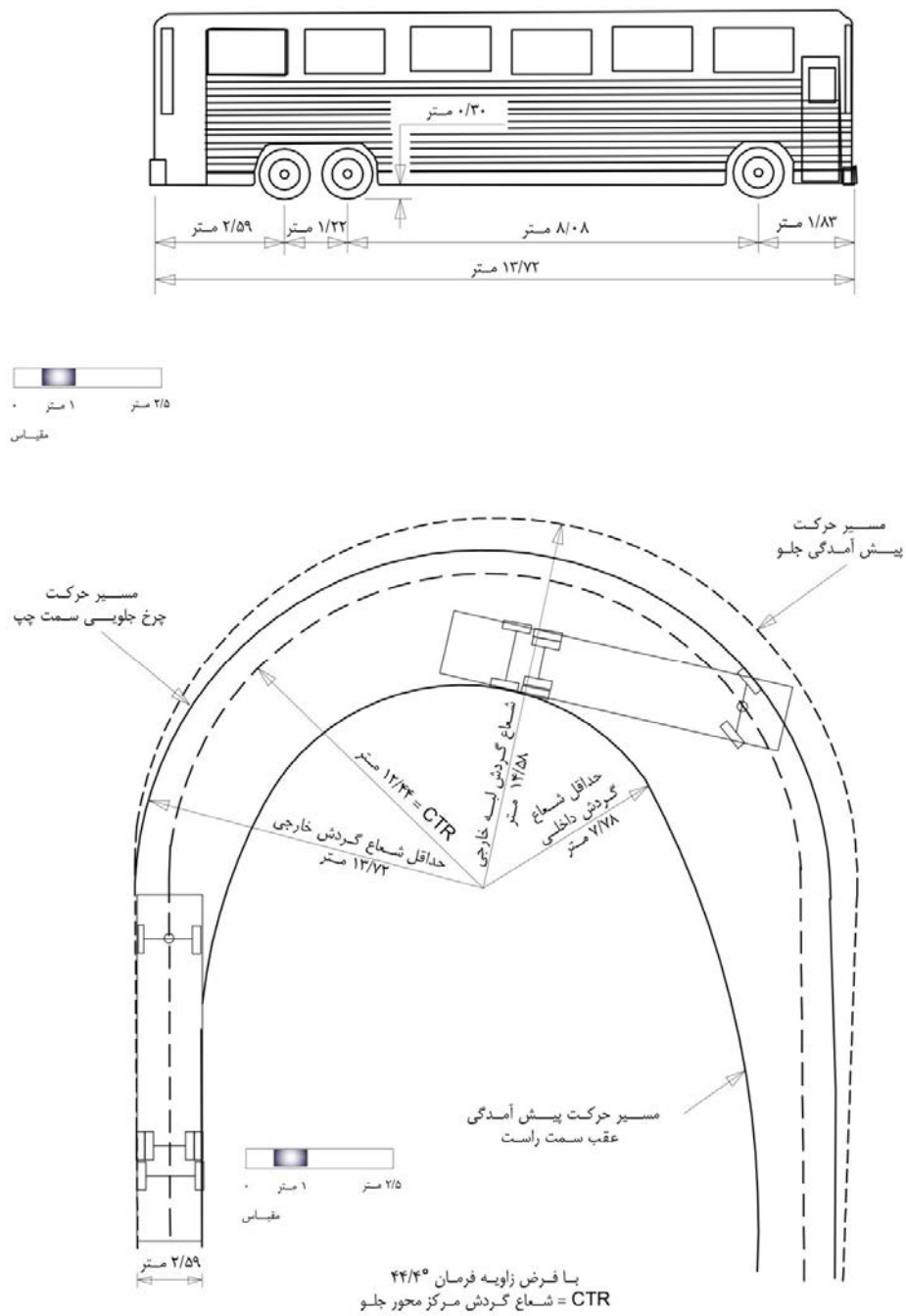
شکل ۴-۳- مشخصات مسیر گردش خودروی طرح، اتوبوس نوع دوم
