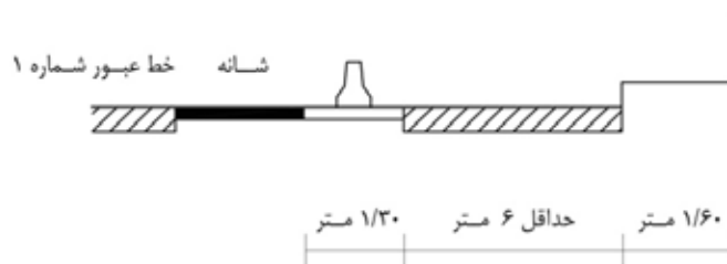
شکل ۴-۱۰ - اندازه و موقعیت ایستگاه اتوبوس
