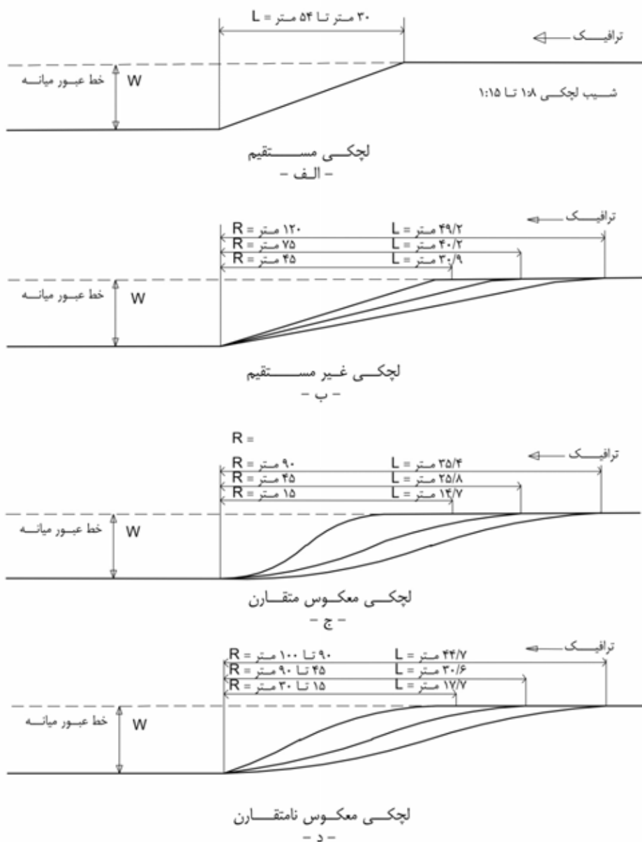
شکل ۸-۴۳- طرح لچکی برای خط کمکی
