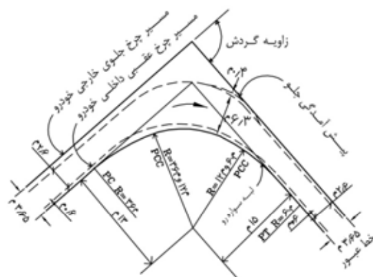
قوس مرکب سه مرکزی با شعاع‌های ۳۶ متر - ۱۲ متر - ۶۰ متر و عقب نشینی ۳۱ متر
