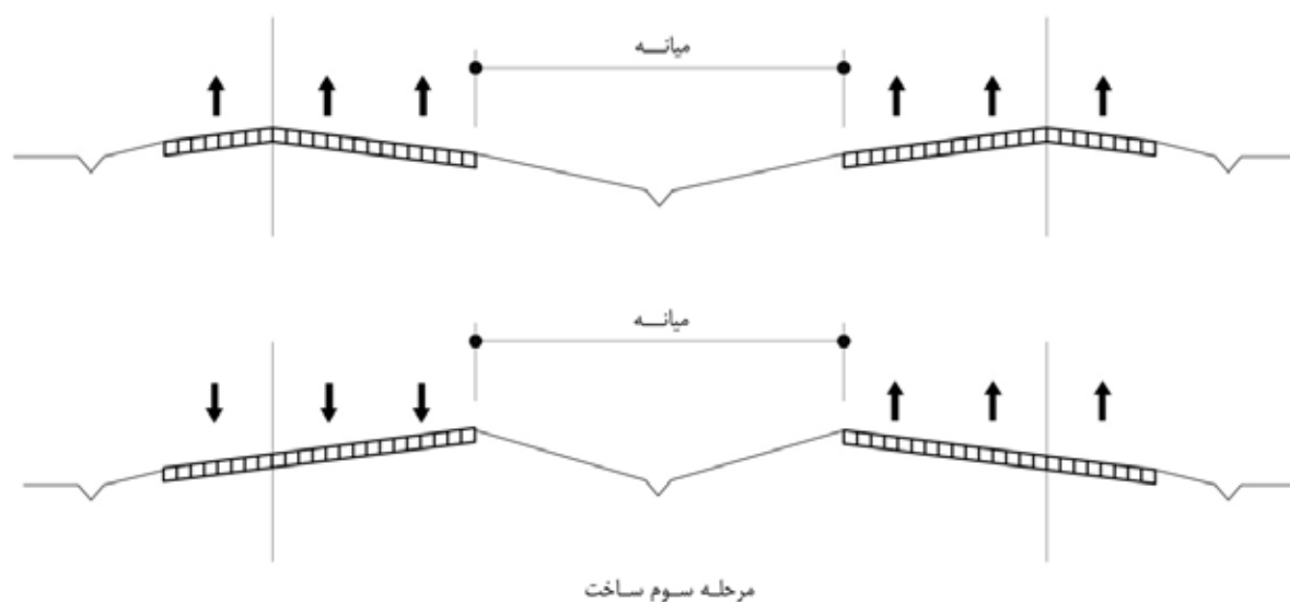
شکل ۴-۸- مرحله سوم ساخت یک راه چند خطه جداشده با میانه عریض
