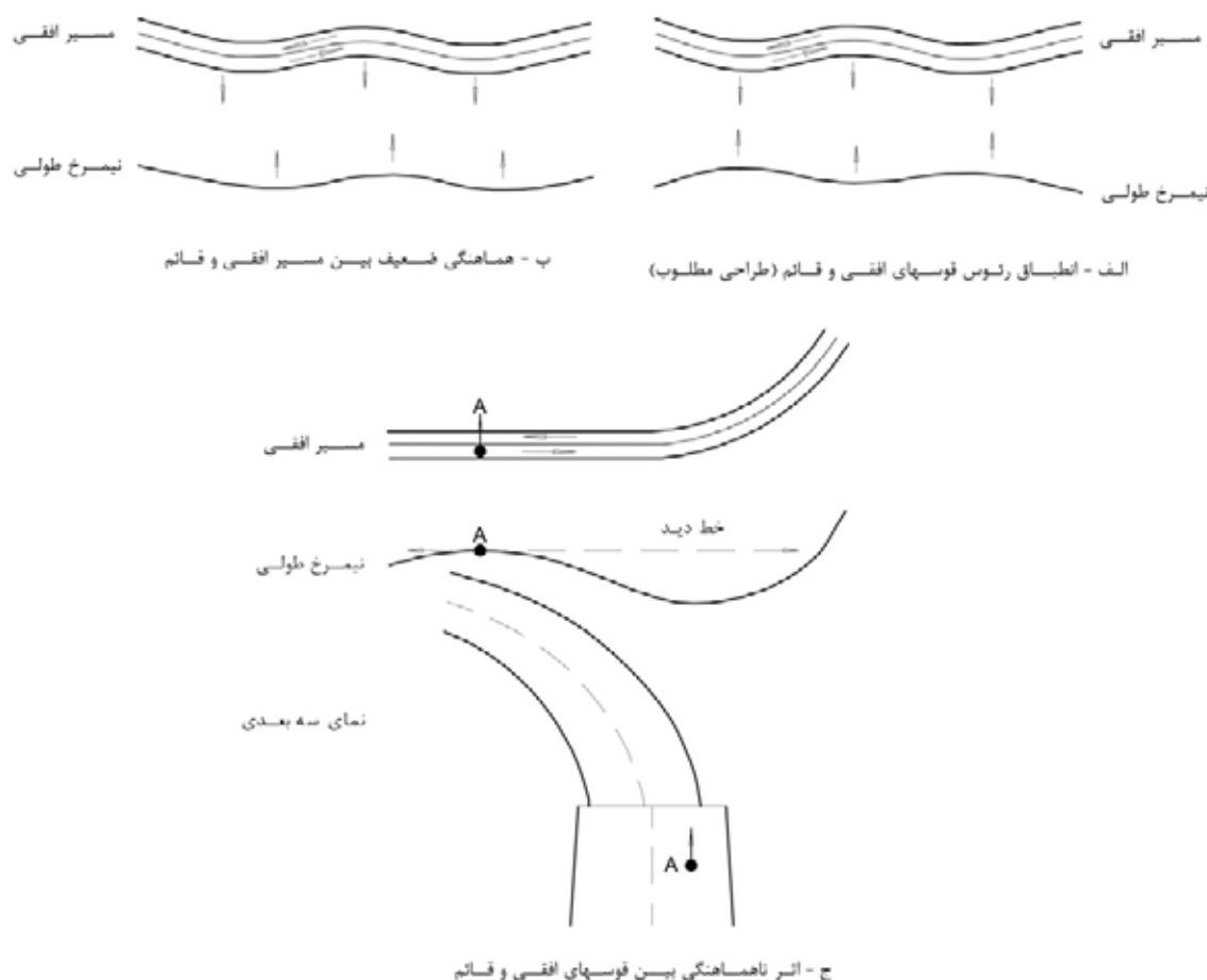
شکل ۵-۱۷- نمونه‌هایی از نحوه هماهنگی پلان و پروفیل طولی راه
