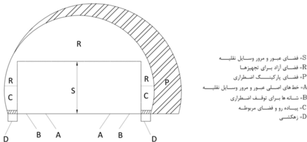
شکل ۶-۲۰- مقطع تونل به همراه پیاده‌روها، شانه‌ها، زهکشی و فضای ویژه توقف‌گاه (پارکینگ) اضطراری
