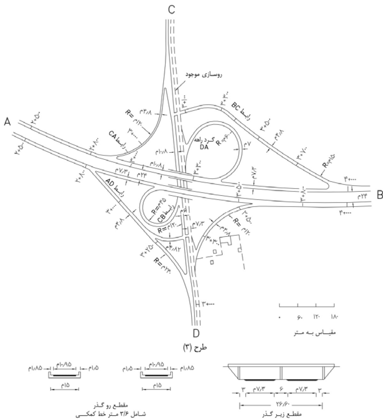
شکل ۹-۳۳- نمونه طرح اولیه تبادل
