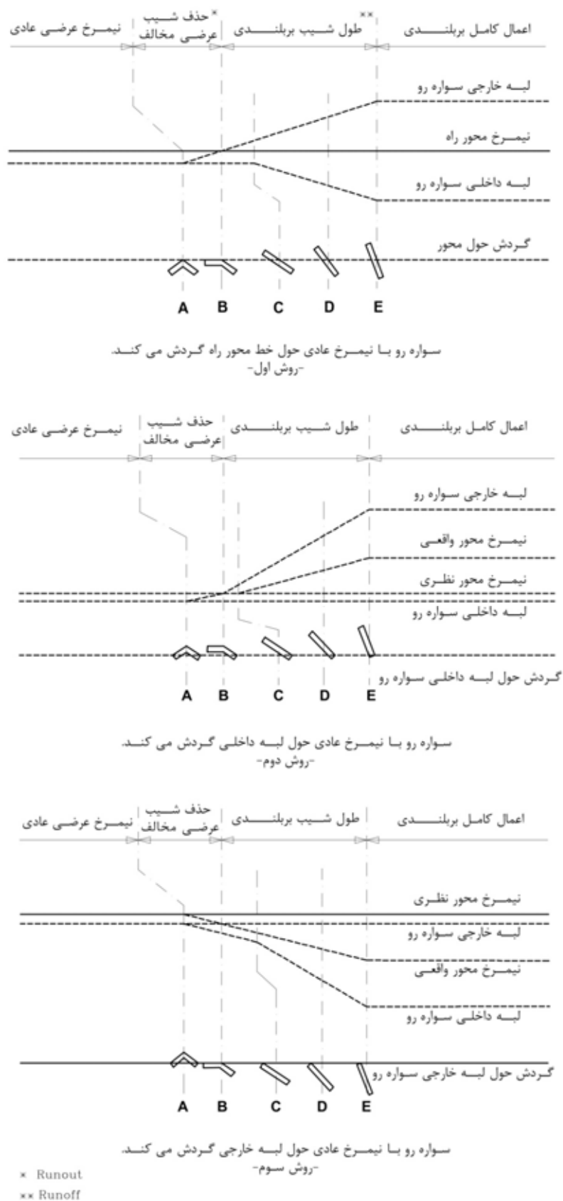
شکل ۵-۵- انواع دوران برپلندی
