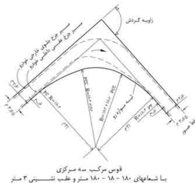
شکل ۸-۲۳- حداقل مسیر گردش برای کامیون نوع دو
