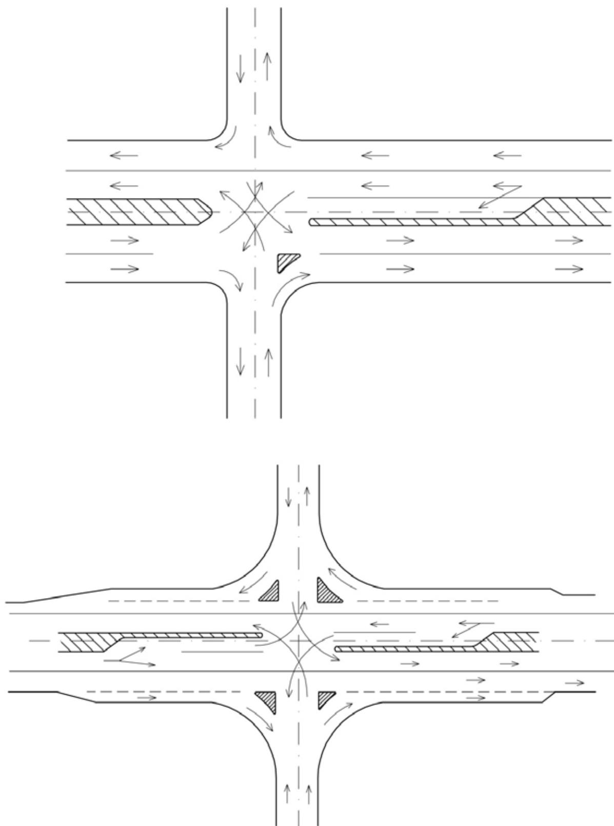
شکل ۸-۱۳- نمونه‌هایی از چهارراه جریان‌بندی شده
