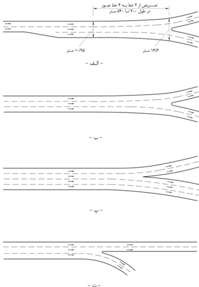
شکل ۹-۲۹- حالت‌های متداول خروجی‌های چند شاخه‌ای
