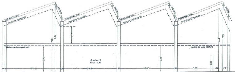
Coupe
