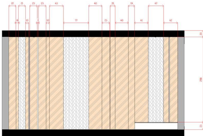
1 Master Bedroom 1 : 25
