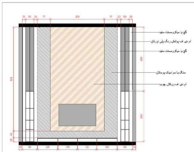
1 Tv wall 1 : 50
