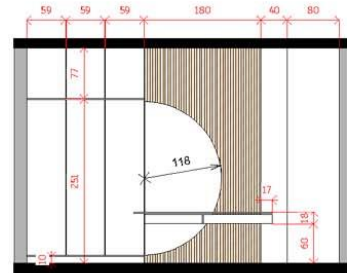
2 Bed Room 2 1 : 50
