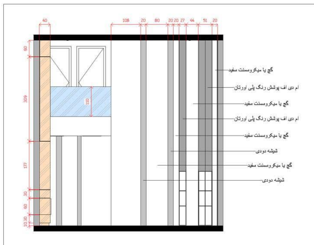
1 Wall 1 : 50
