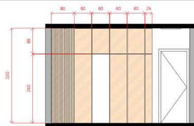
1 Bed Room 1 1 : 50
