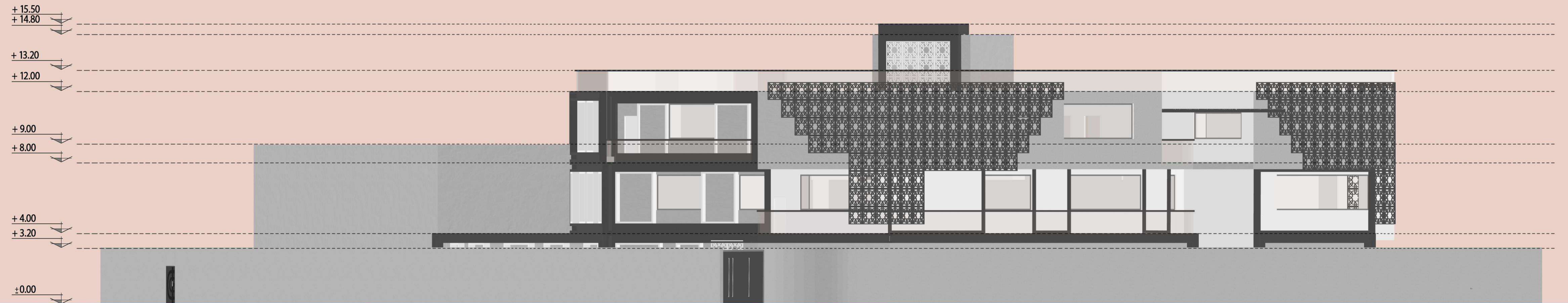
نمای جنوبی
