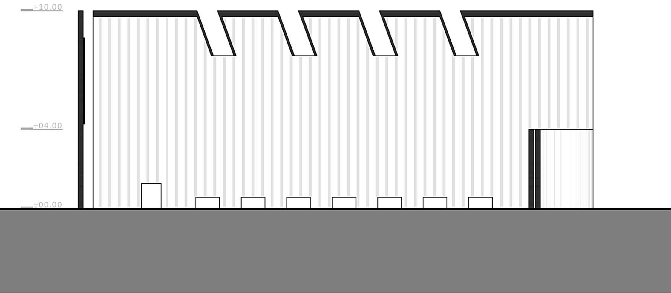
Section A-A
