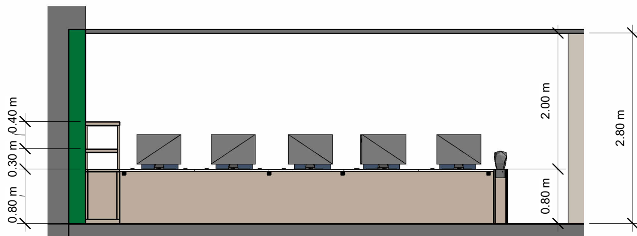
3 برش 2 1 : 50
