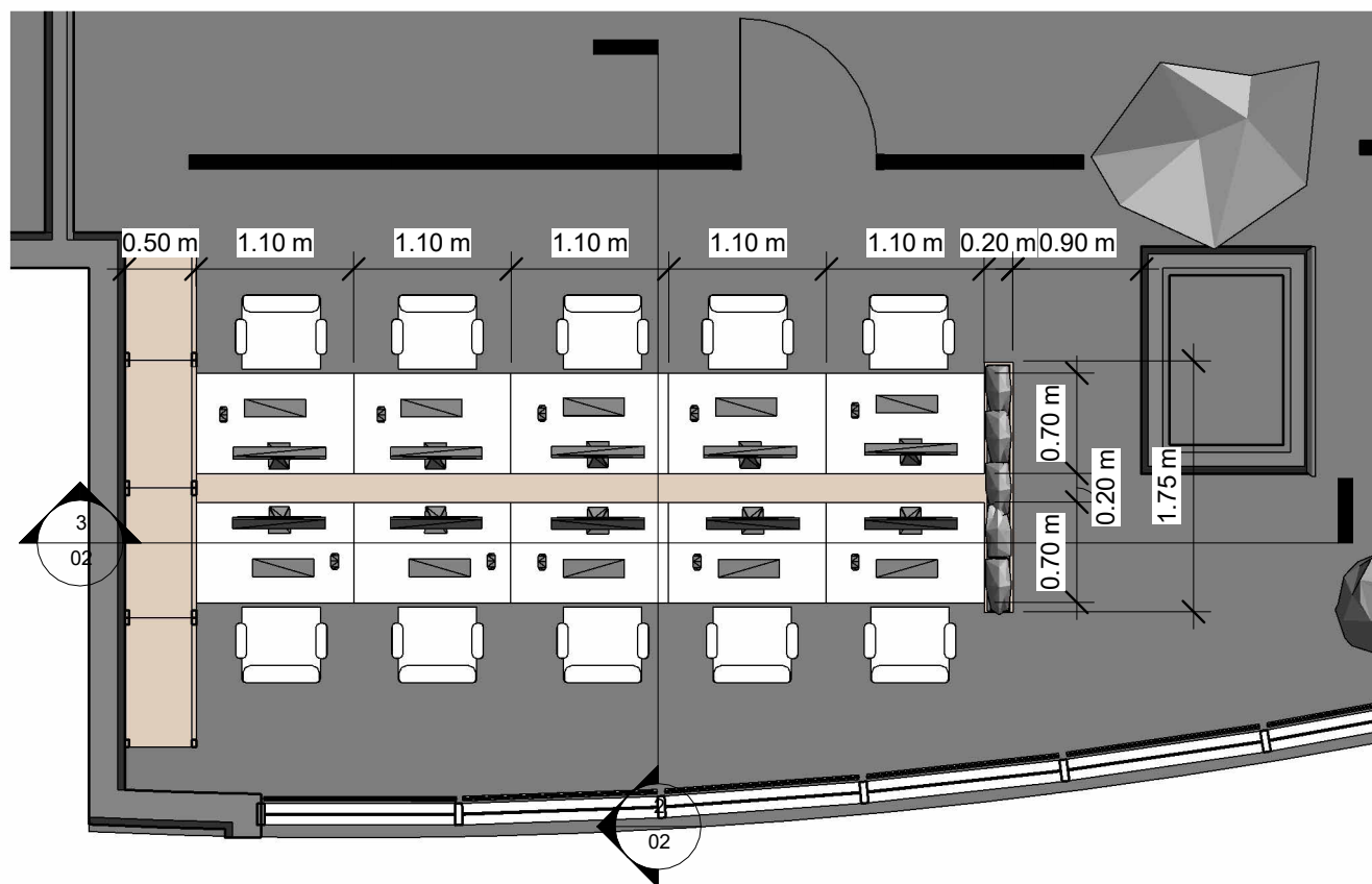
4 اتاق بازرگانی 1 : 50
