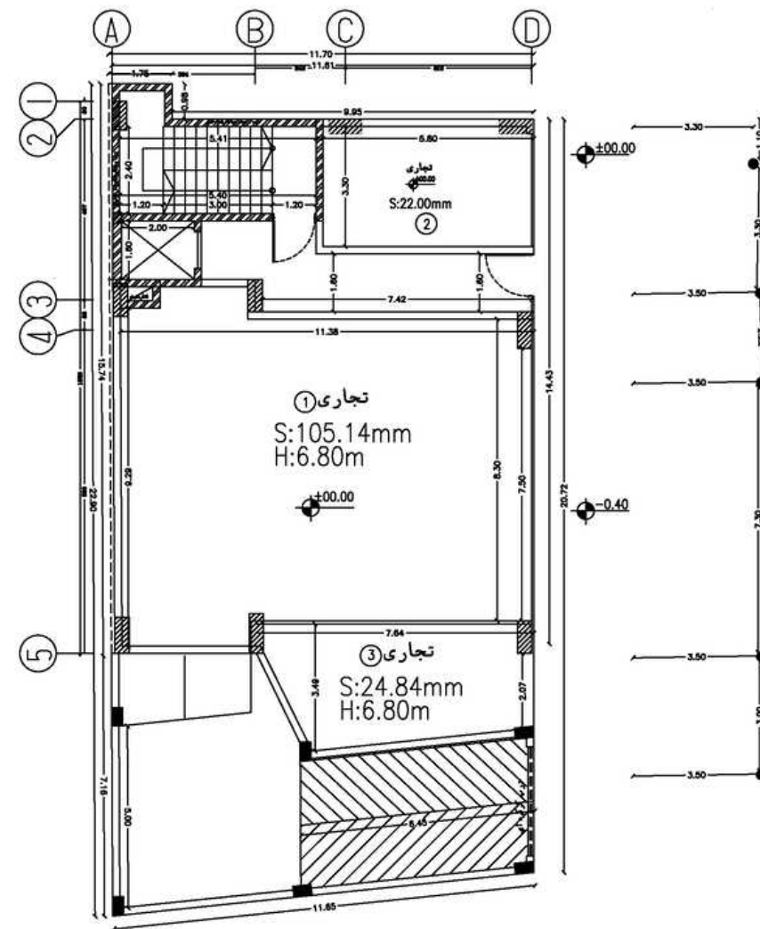
پلان طبقه همکف
