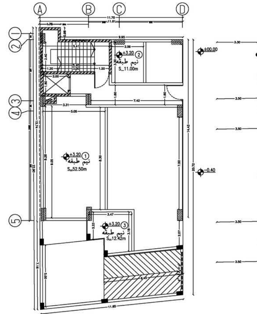
پلان نیم طبقه
