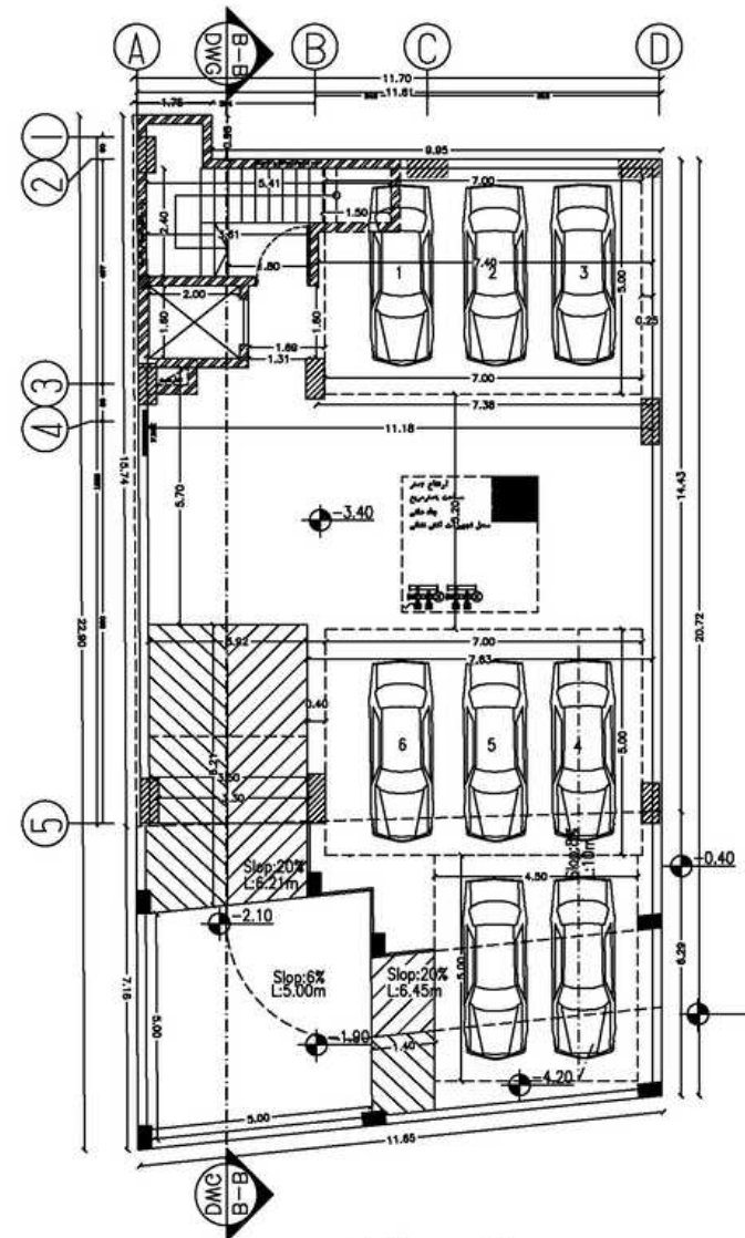
پلان طبقه ۱-
