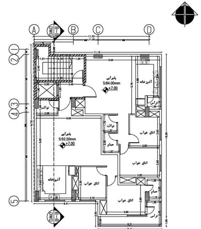
پلان طبقه ۱
