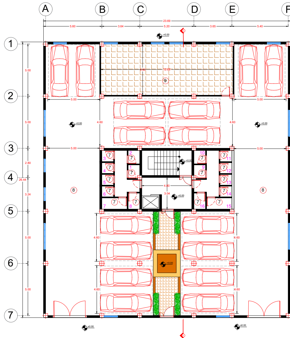
پلان اندازه گذاری طبقه همکف (تیب ۱)
