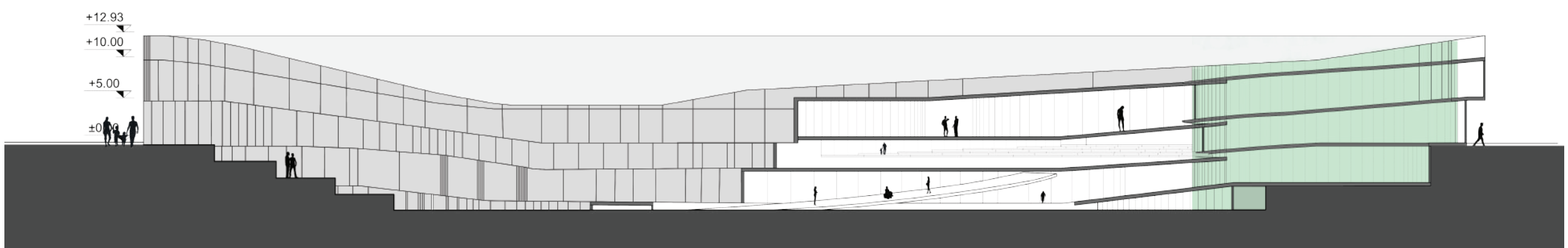
برش B- B
