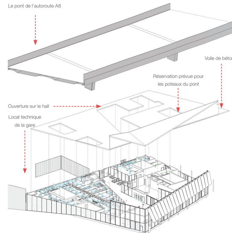
Vue isométrique du bâtiment voyageur et l'autoroute
