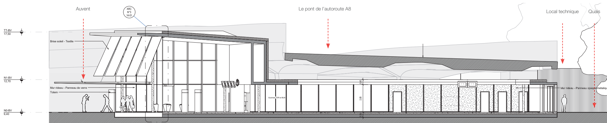
Coupe transversale du bâtiment voyageur
