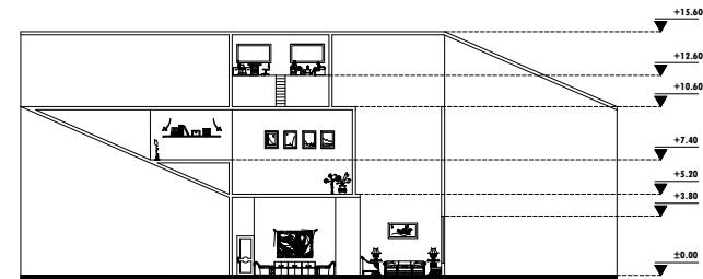
section B-02 scale: 1:100
