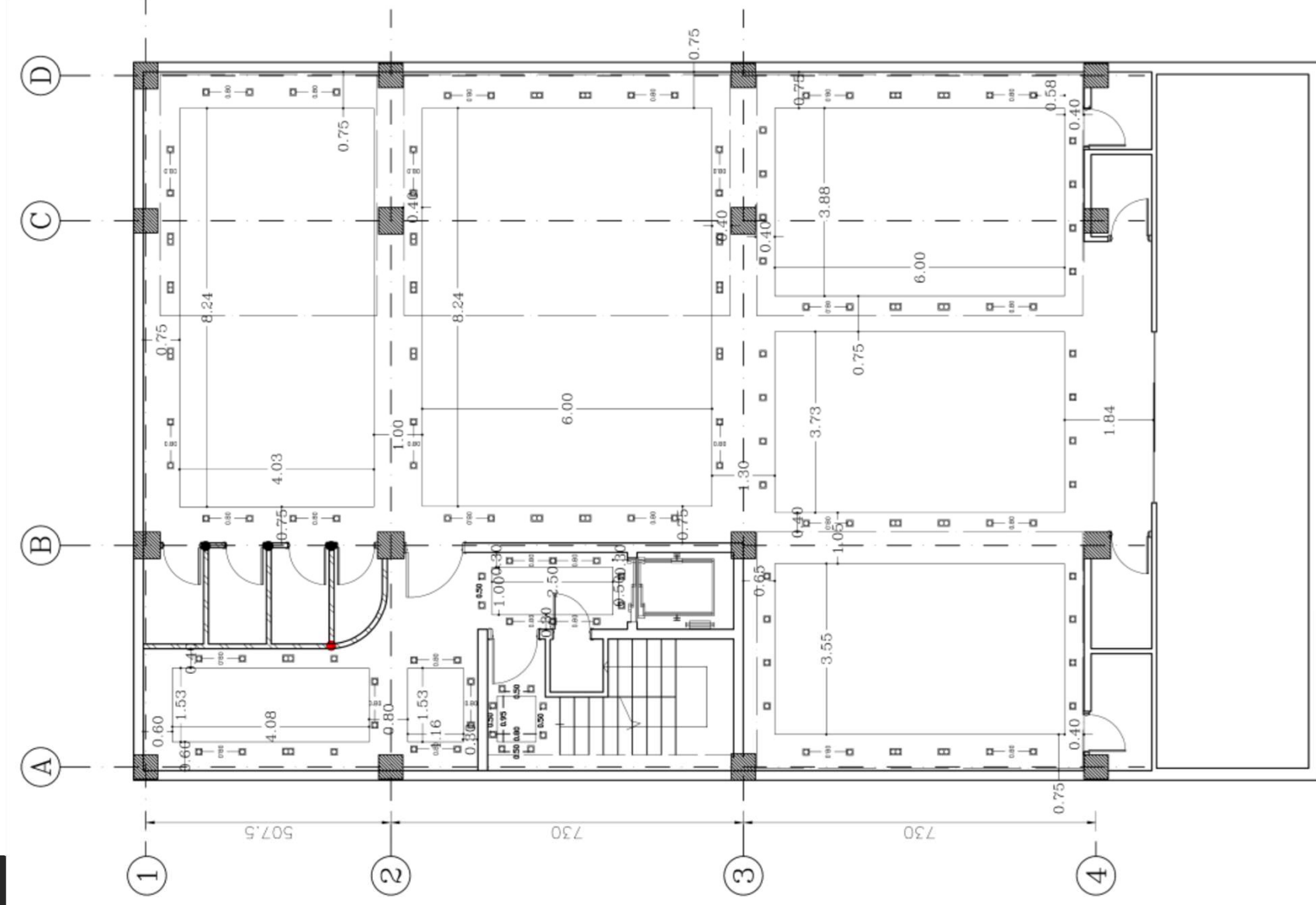
نقشه سقف و نورپردازی پارکینگ و لابی
