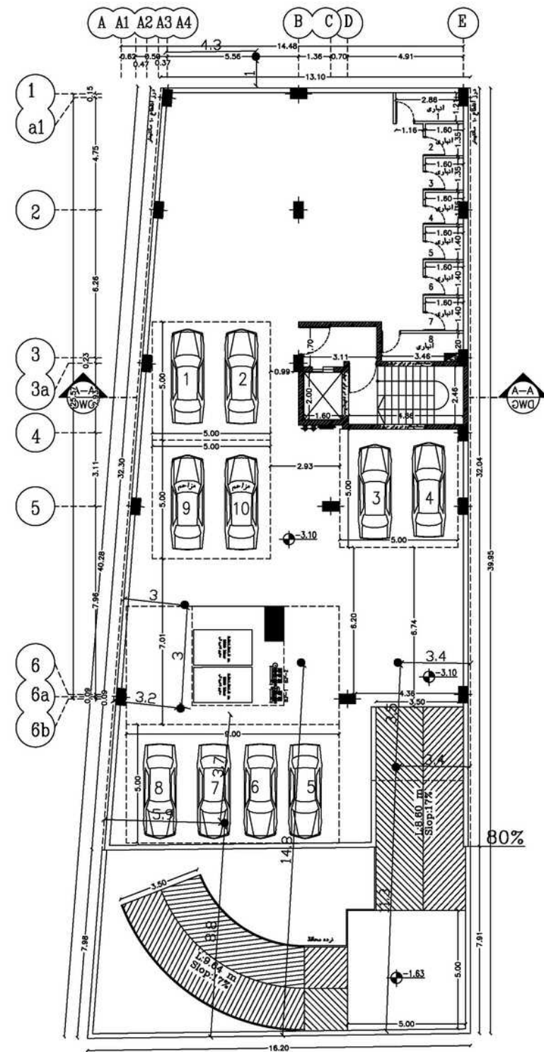
پلان طبقه ۱- SC:1/100
