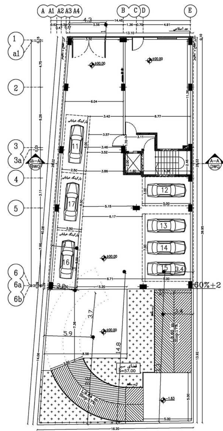
پلان طبقه همکف SC:1/100
