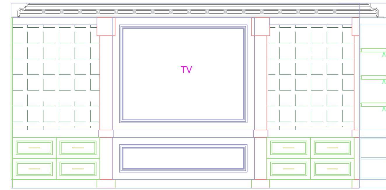
A-A VIEW
