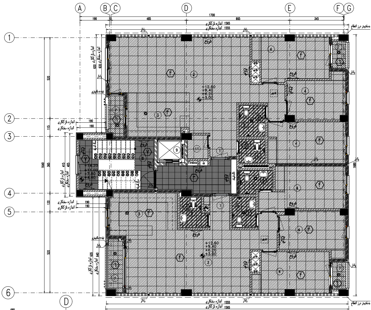
پلان کفسازی تپ طبقات
