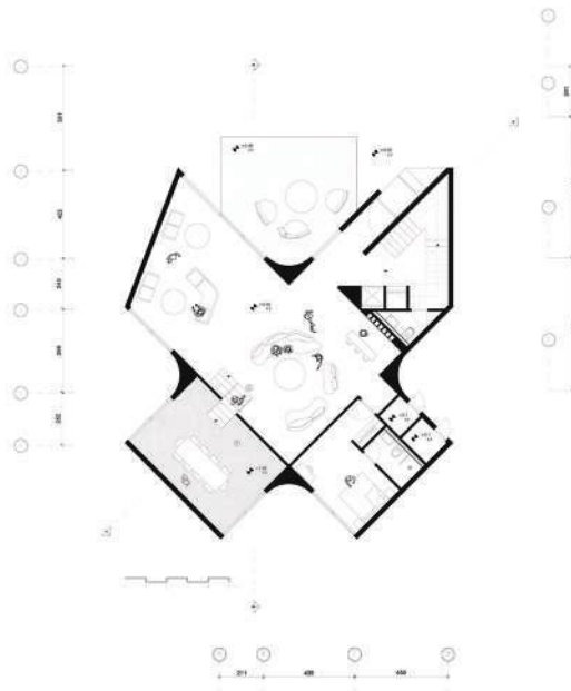
ویلای آوانگارد پلان نیم طبقه
