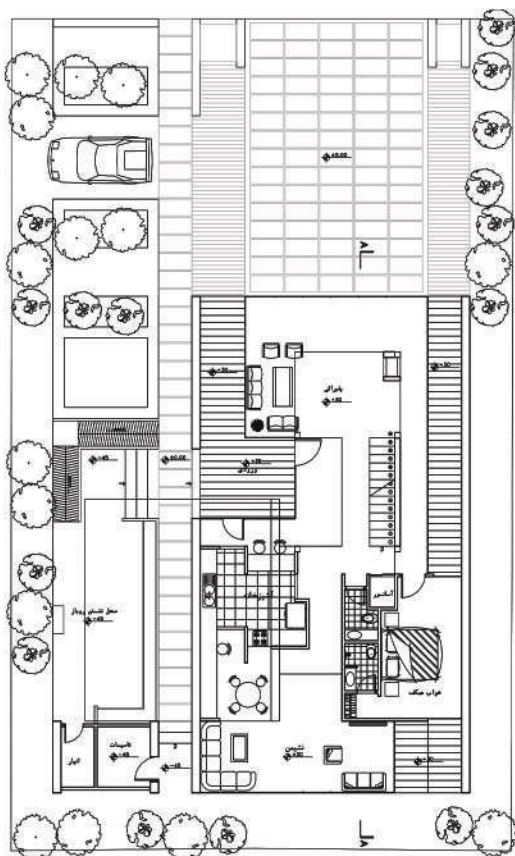
پلان طبقه همکف
