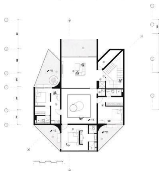
ویلای آوانگارد پلان طبقه اول
