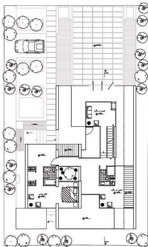
پلان مبلان میان طبقه
