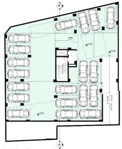
پلان میلمان زیرزمین 2-
