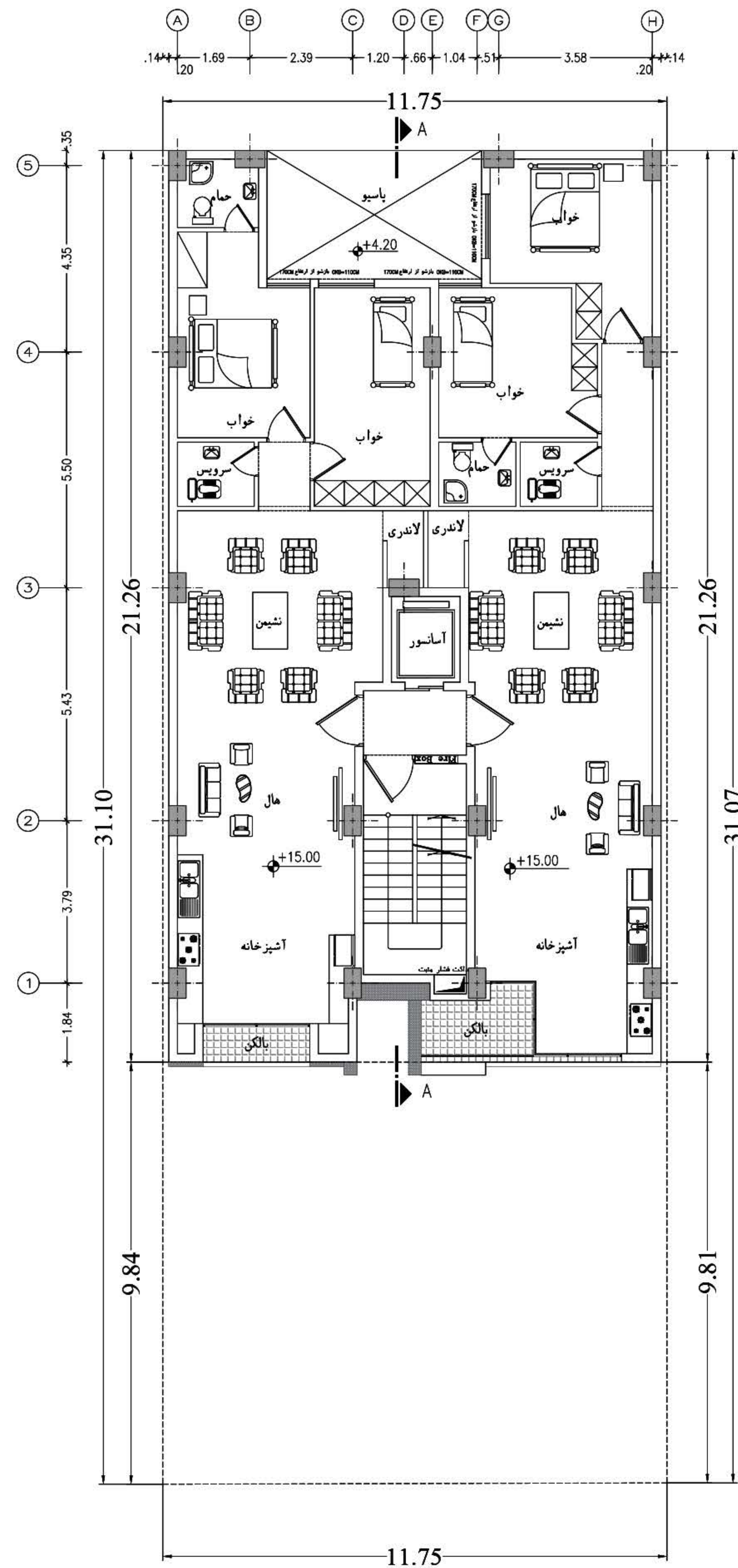
پلان طبقه چهارم
