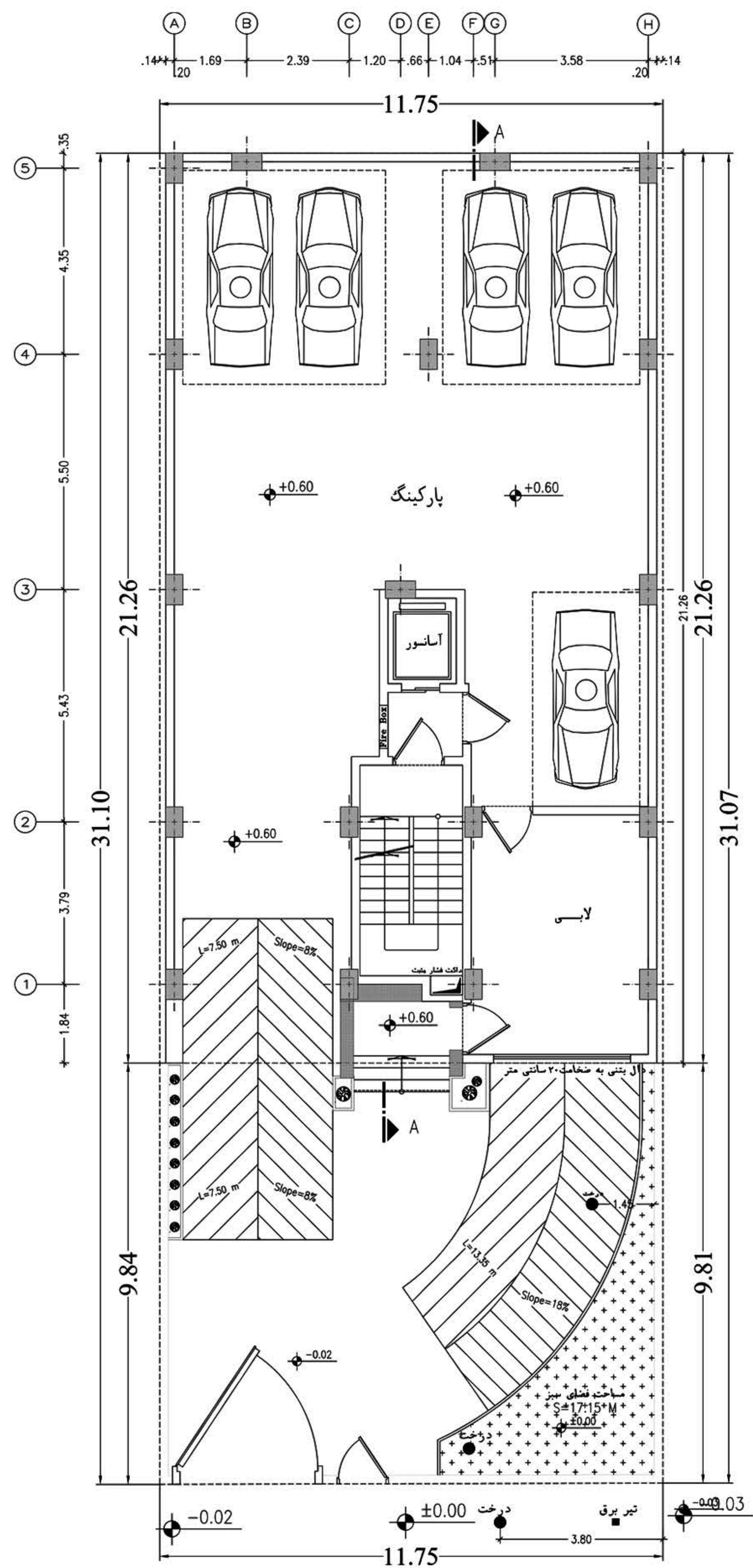
پلان همگف
