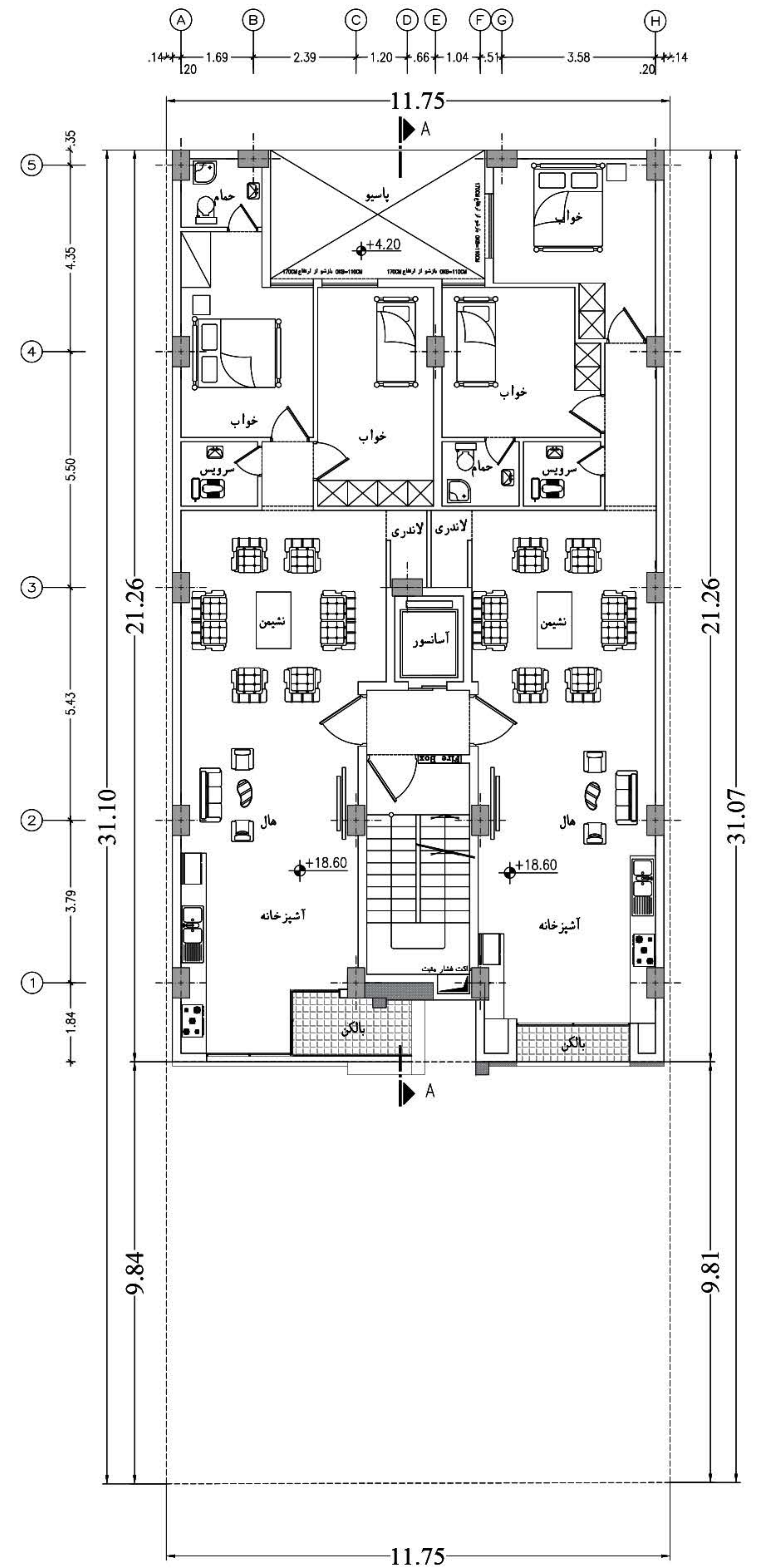
پلان طبقه پنجم
