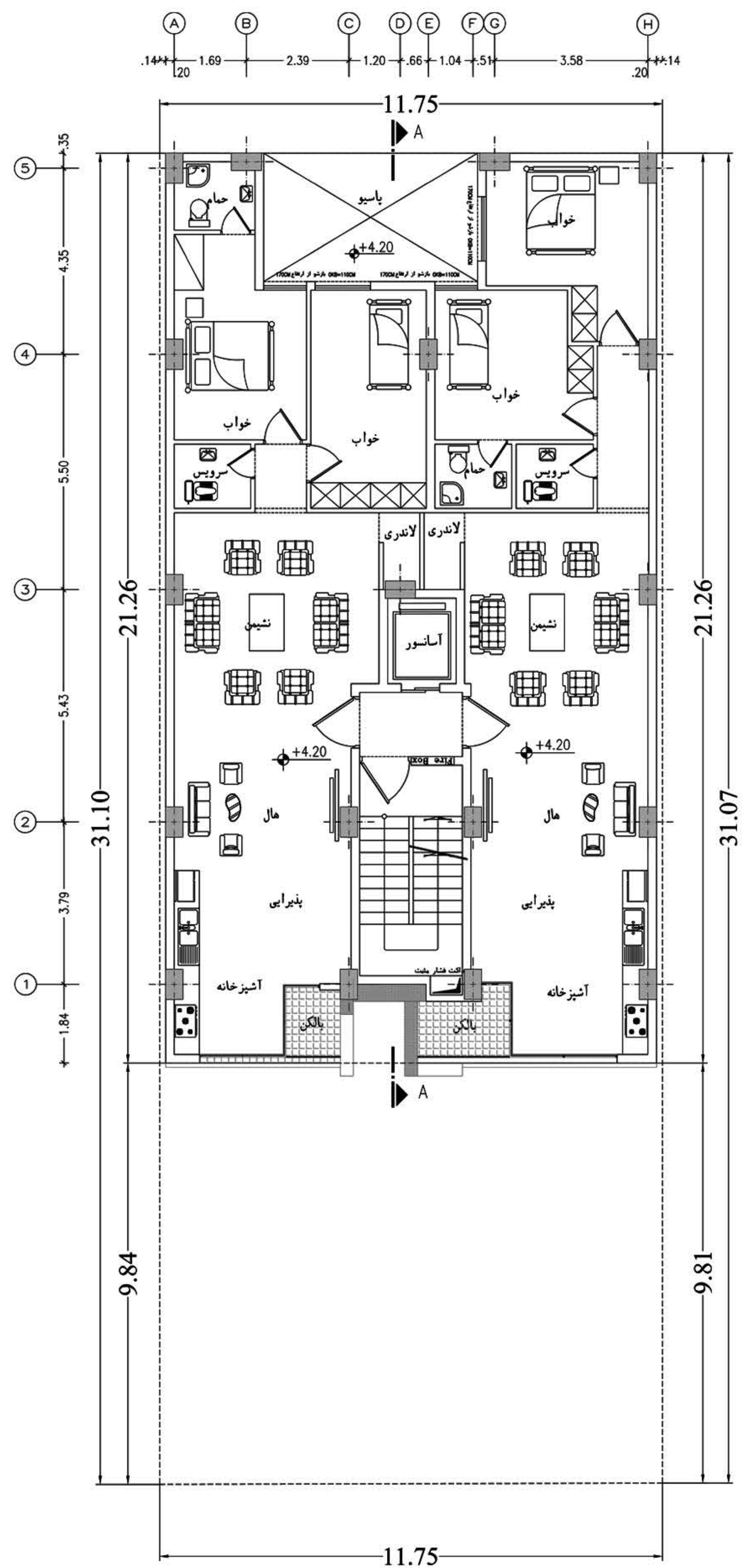
پلان طبقه اول
