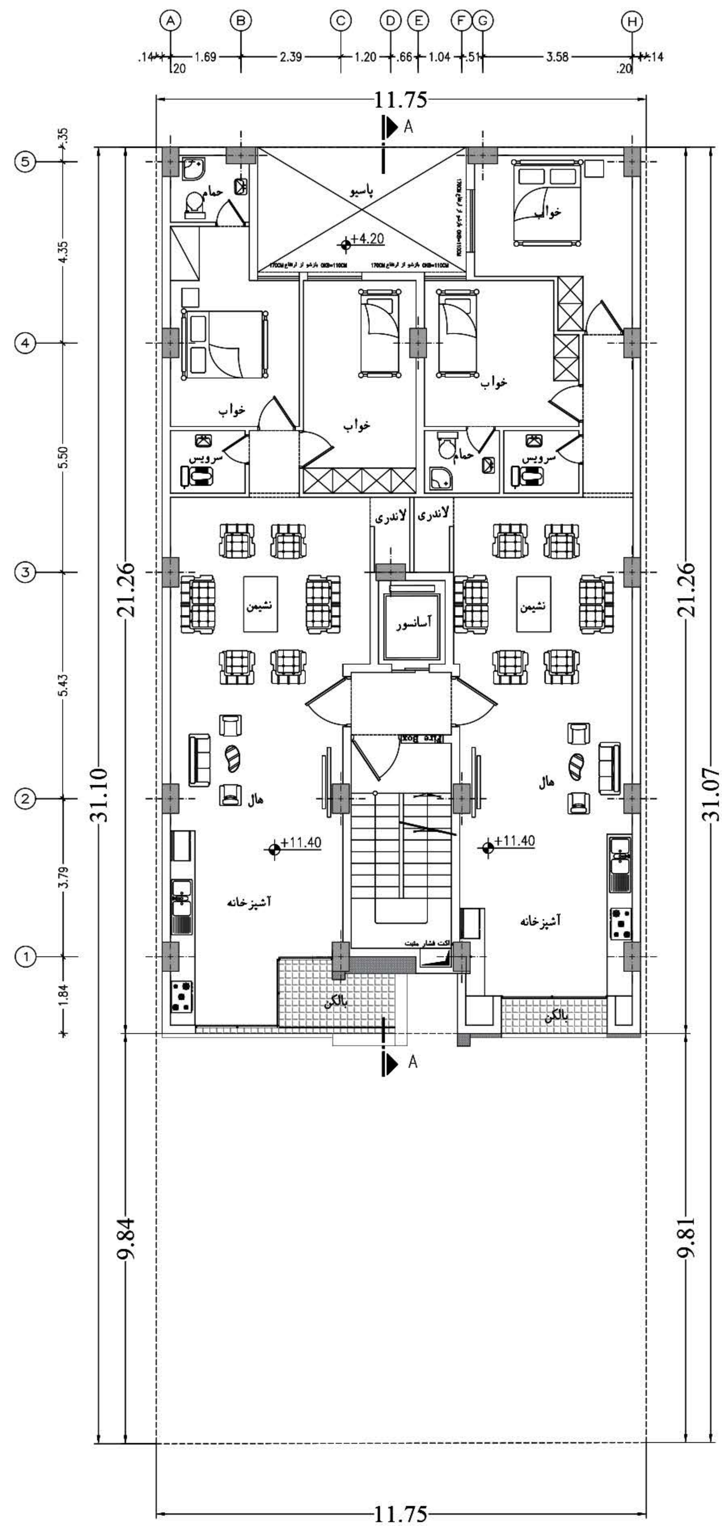
پلان طبقه سوم
