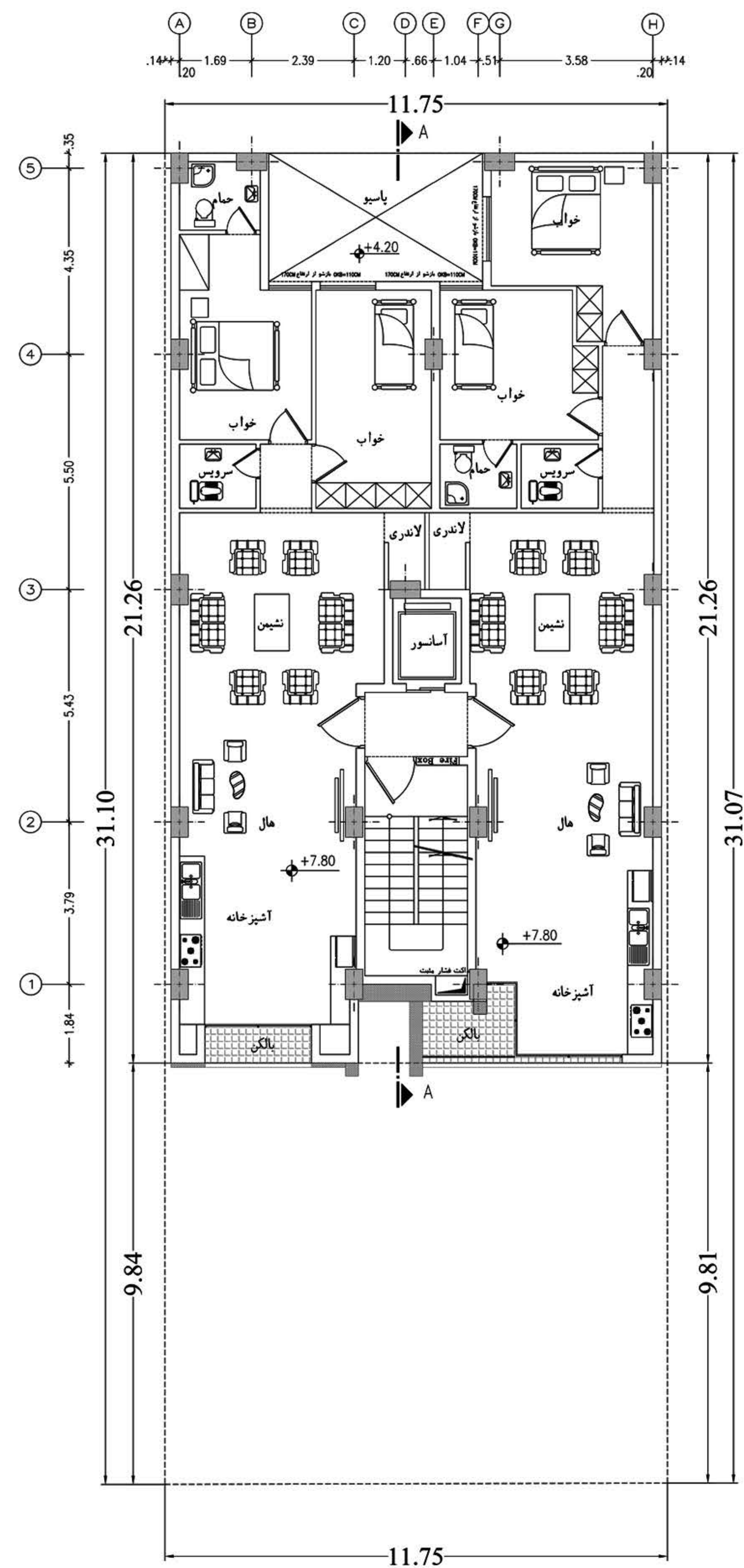
پلان طبقه دوم
