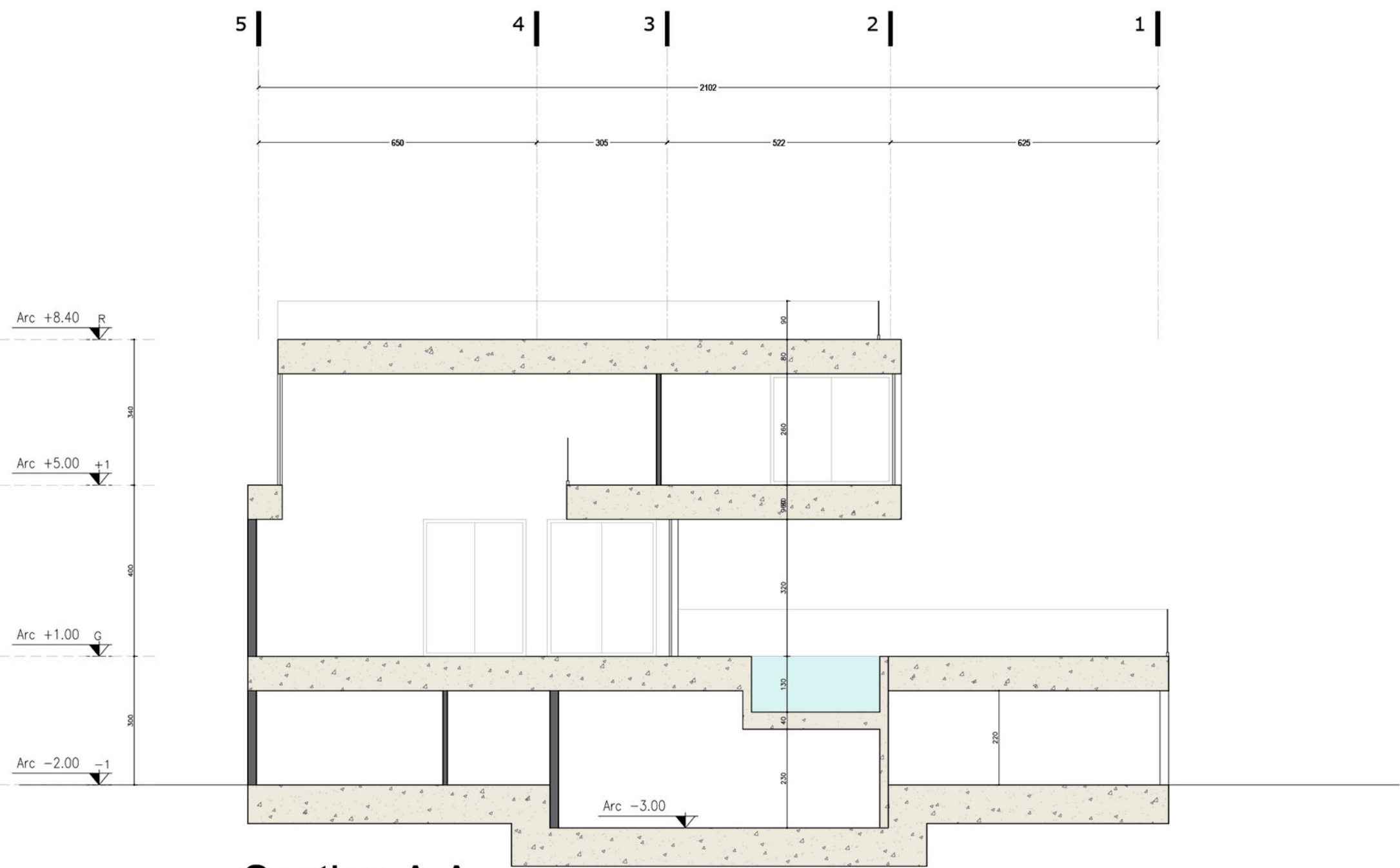
Section A.A
