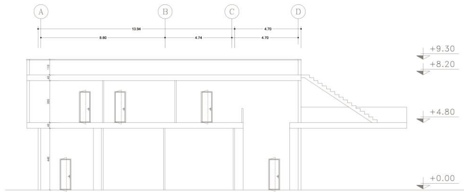
SECTION A-A SC;1:100
