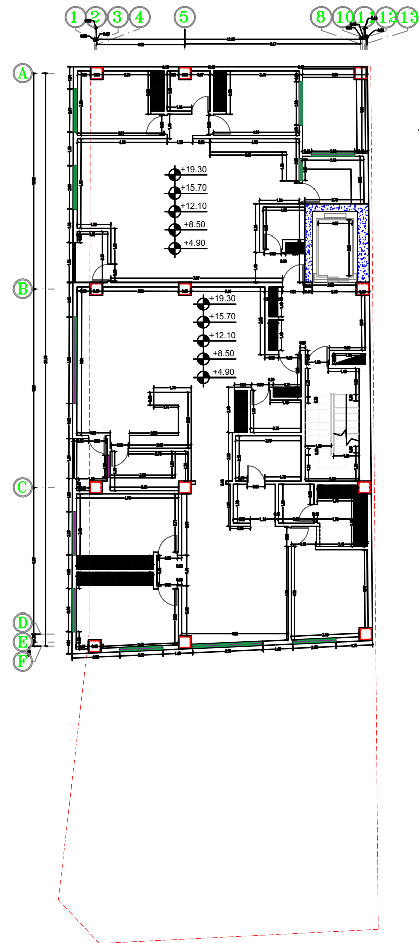
پلان اندازه گذاری تپ طبقات اول تا پنجم
