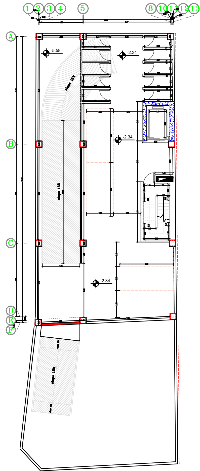
پلان اندازه گذاری زیر زمین اول
