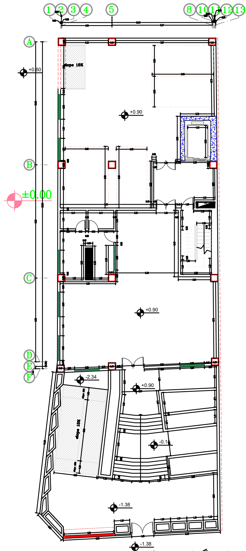
پلان اندازه گذاری همکف
