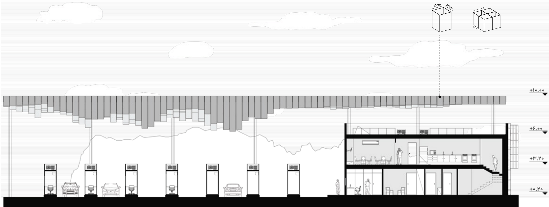
برش معماری دروازه ورودی
