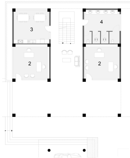
طبقه همکف
