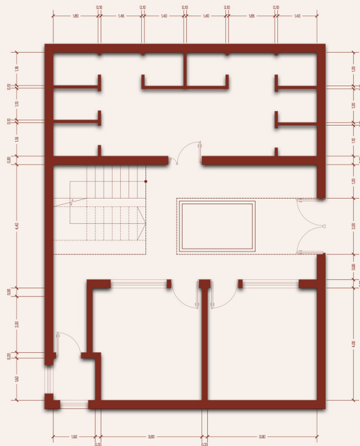
پلان اندازه گذاری همکف ساختمان پرسنل گمرک- شرق
