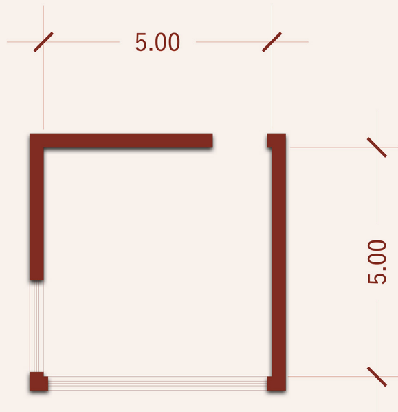
پلان اندازه گذاری نگهبانی
