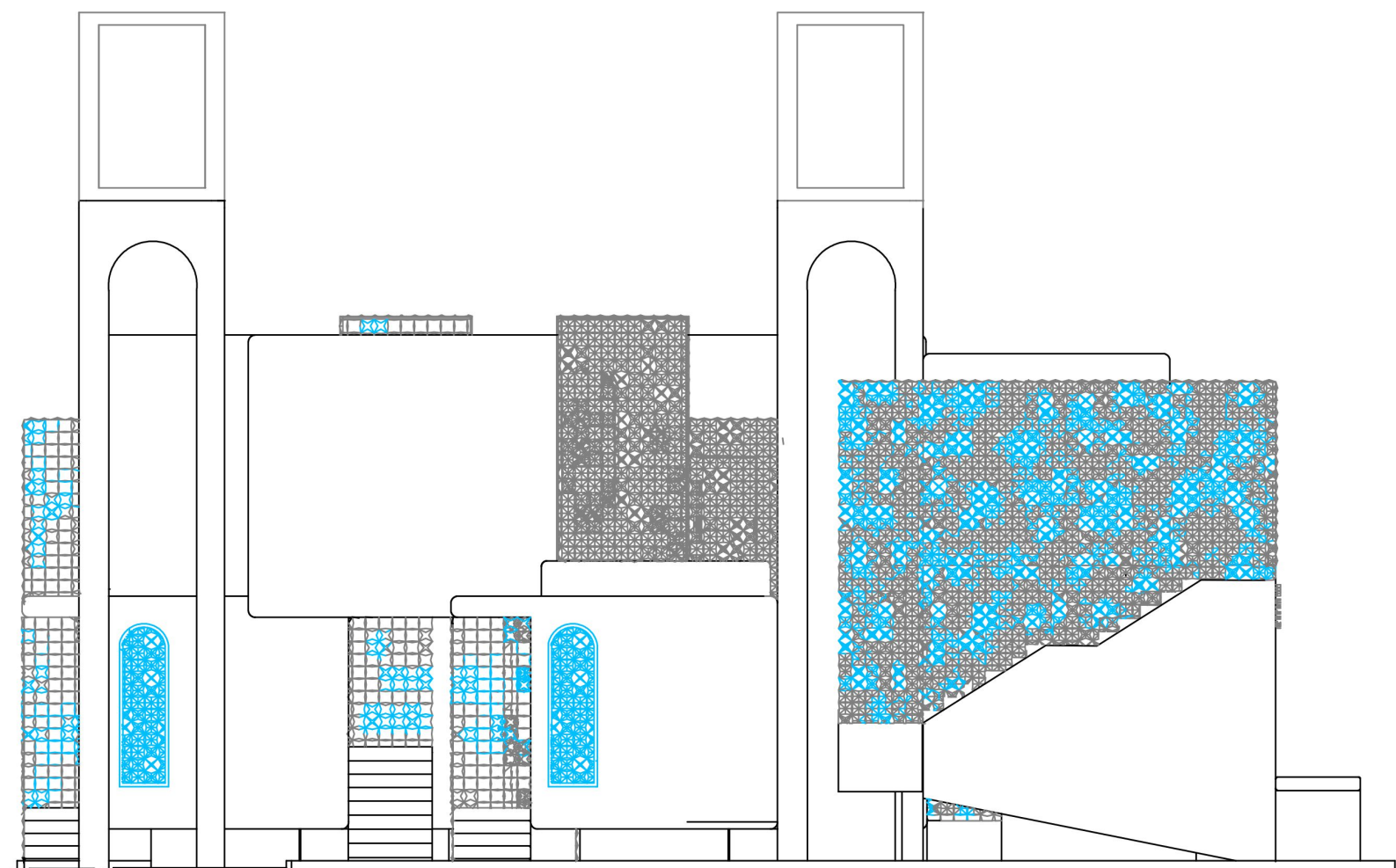
B SECTION B-2 SCALE: 1/100
