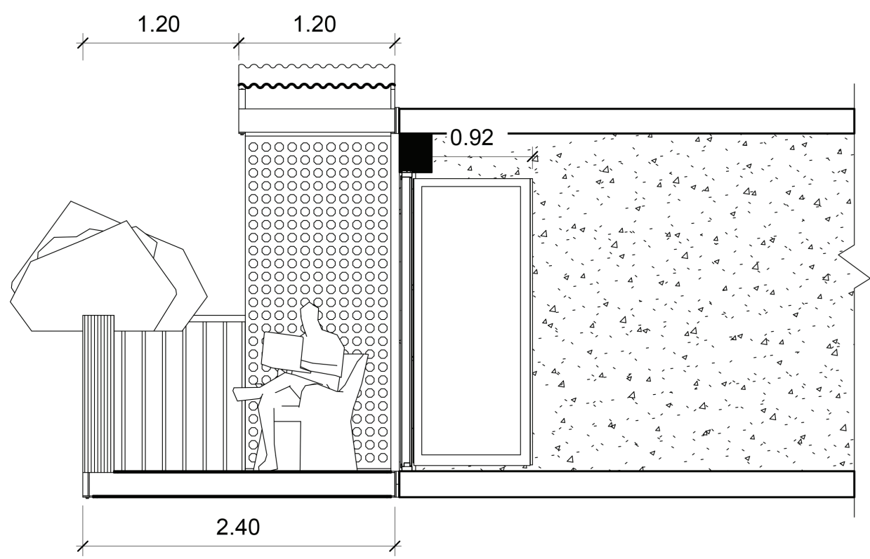
Section A-A
