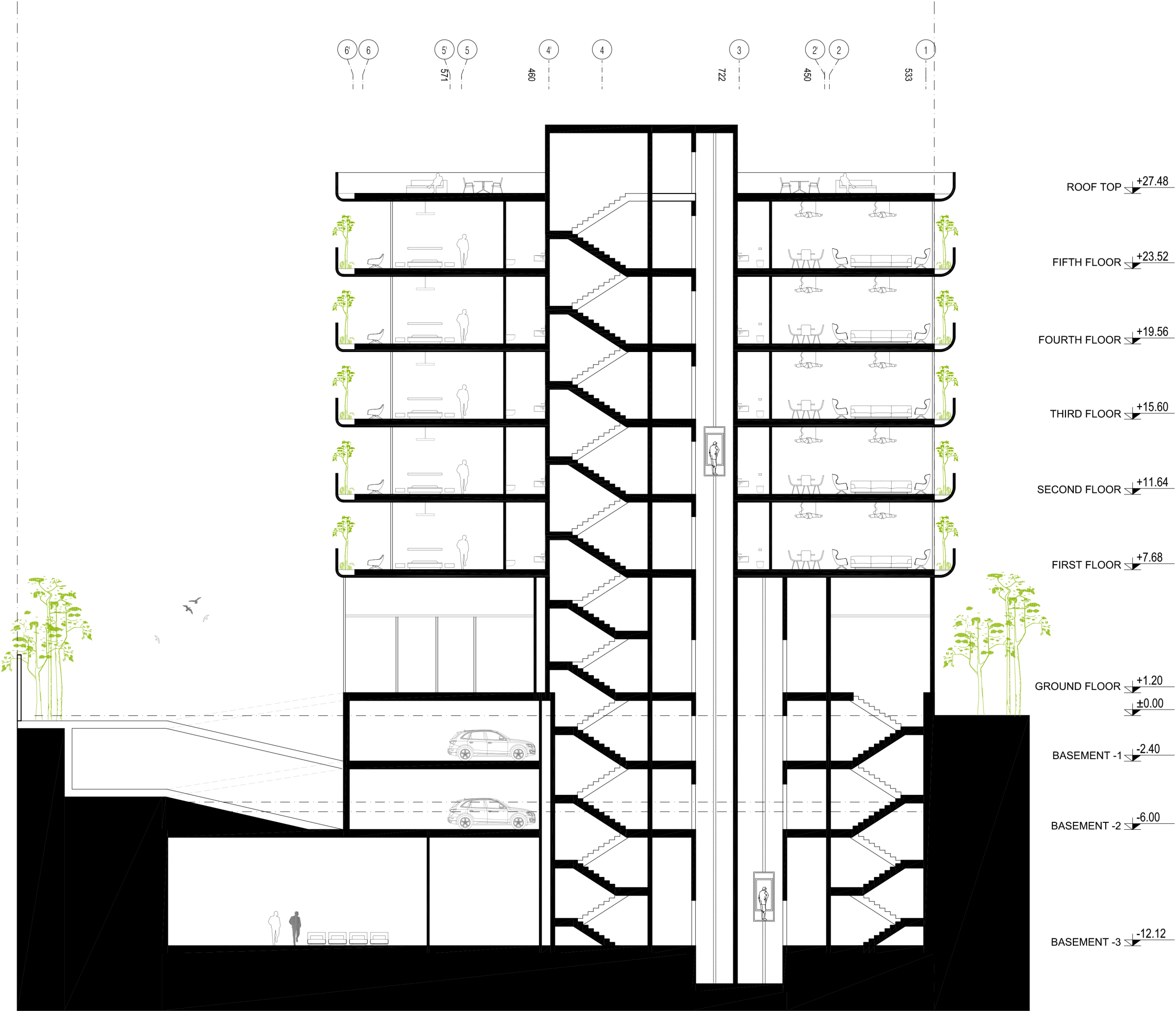
SECTION A-A
