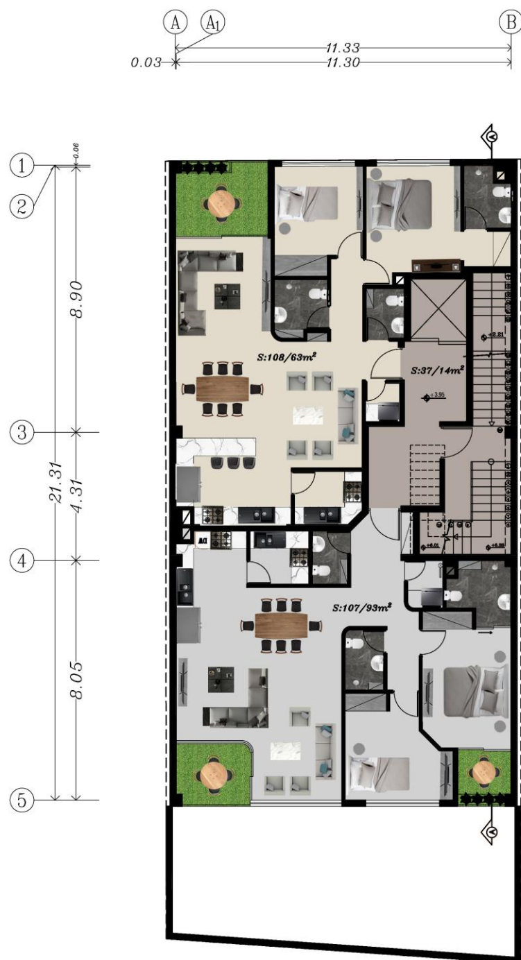
پلان طبقه اول
