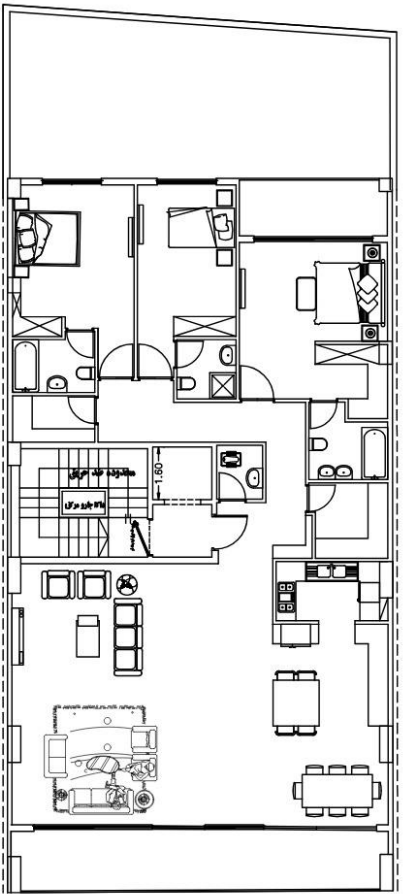
پلان طبقه ۴ و ۵ ۱/۲۰۰
