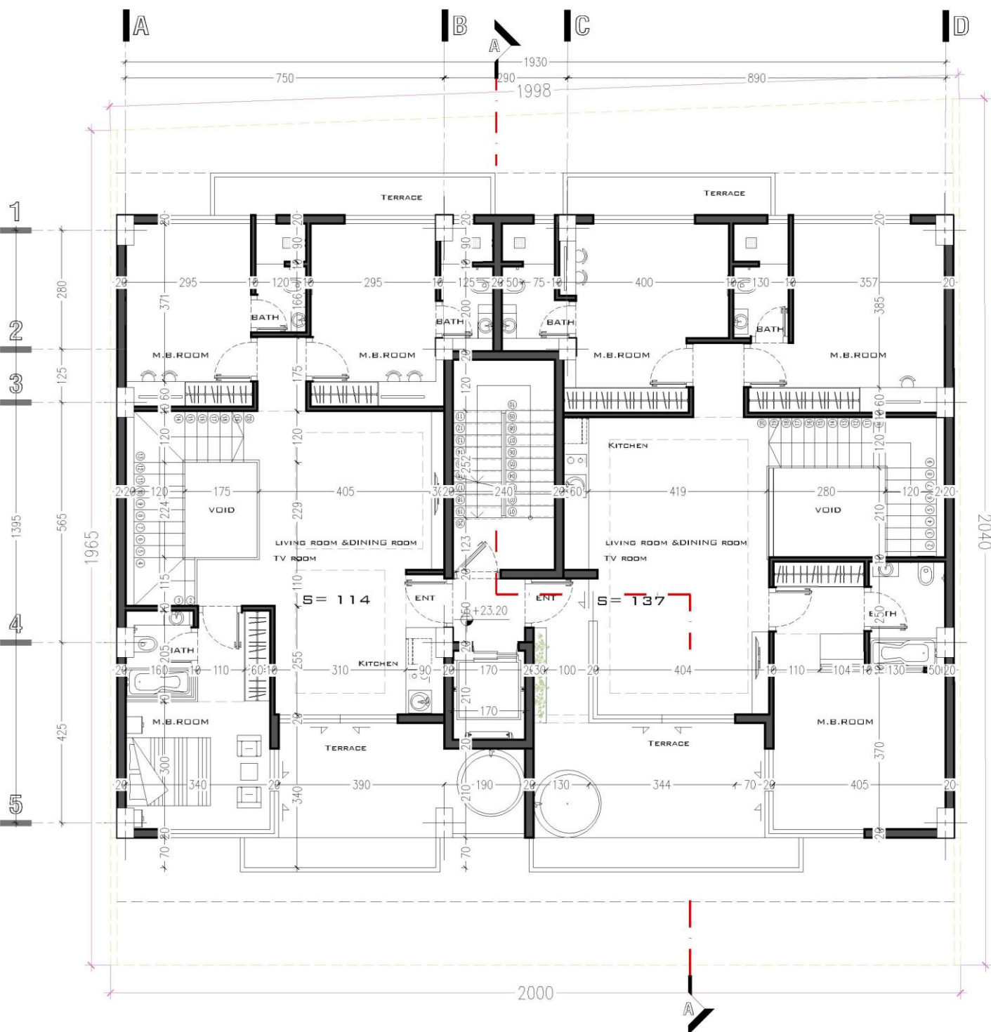
پلان طبقه ۸ اندازه گذاری
