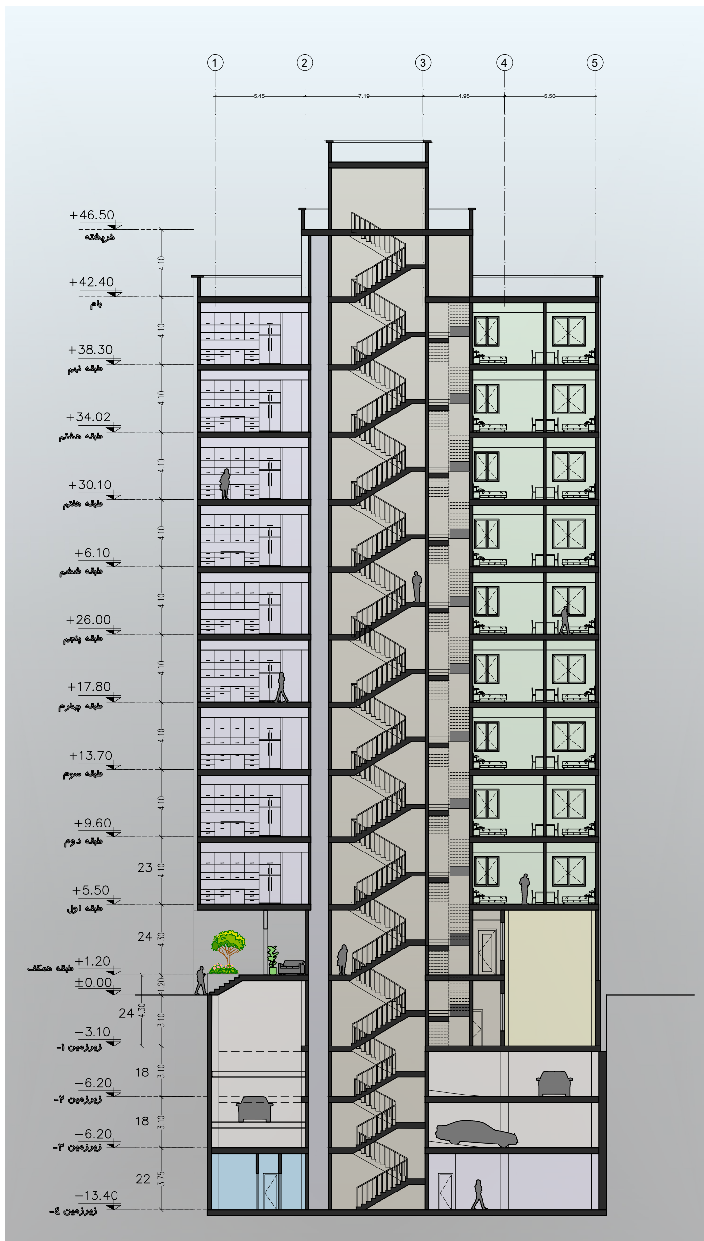
دیاگرام ارتفاعی طبقات
