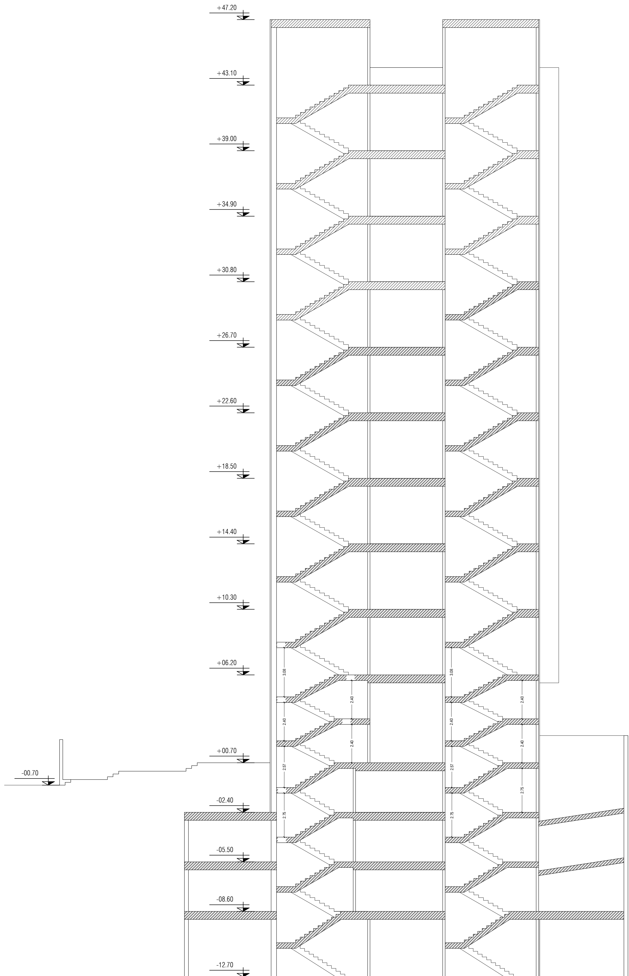
SECTION:A-A
