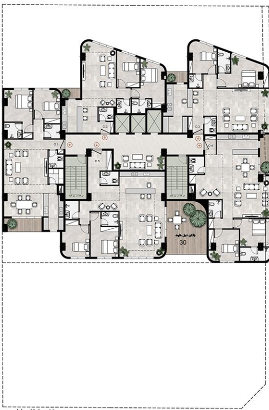
پلان طبقات اول دوم پنجم و ششم و هفتم
