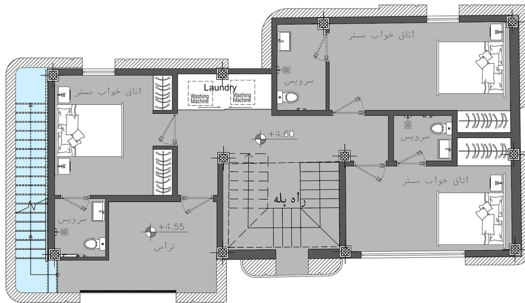
پلان مبلمان طبقه اول
