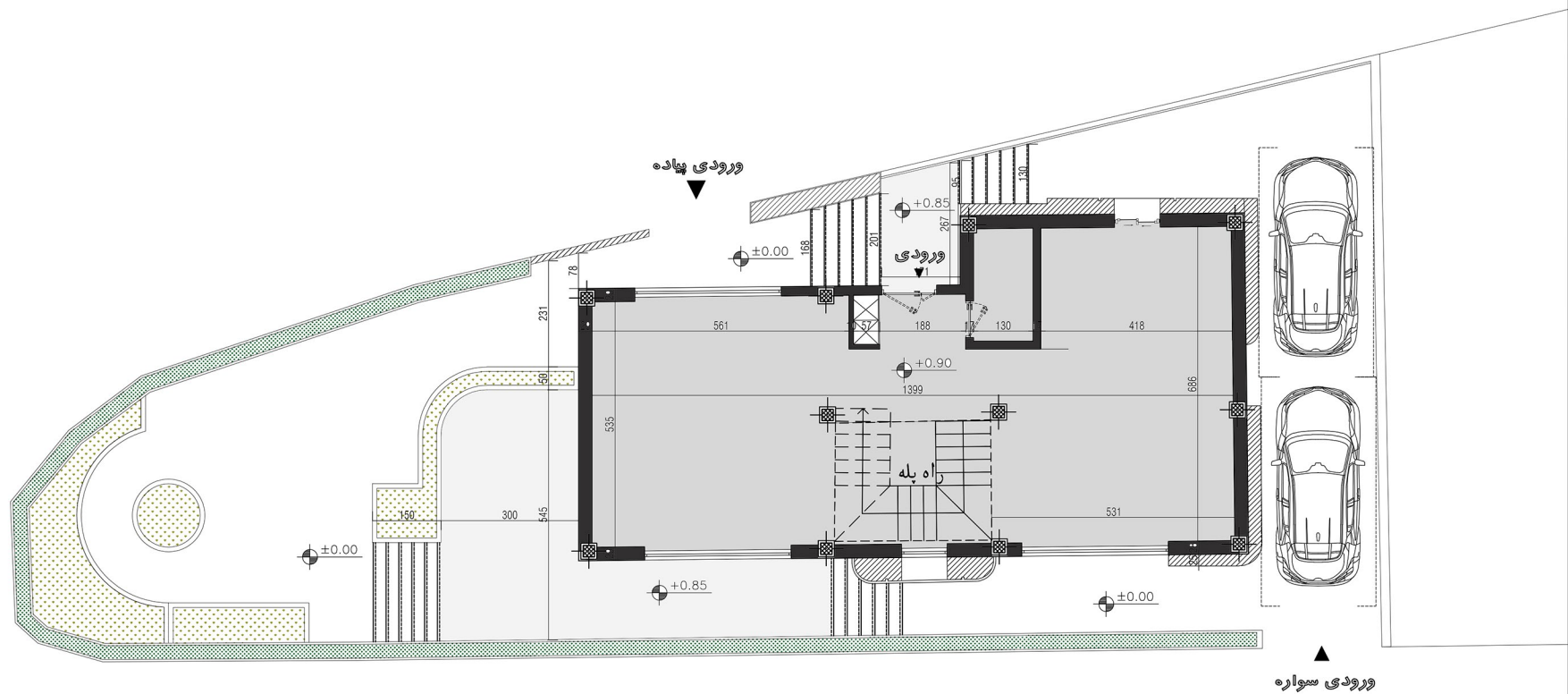
پلان اندازه گذاری طبقه همکف
