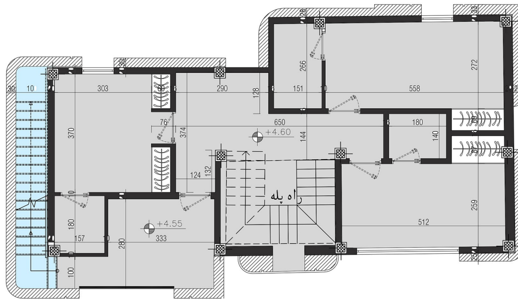
پلان اندازه گذاری طبقه اول
