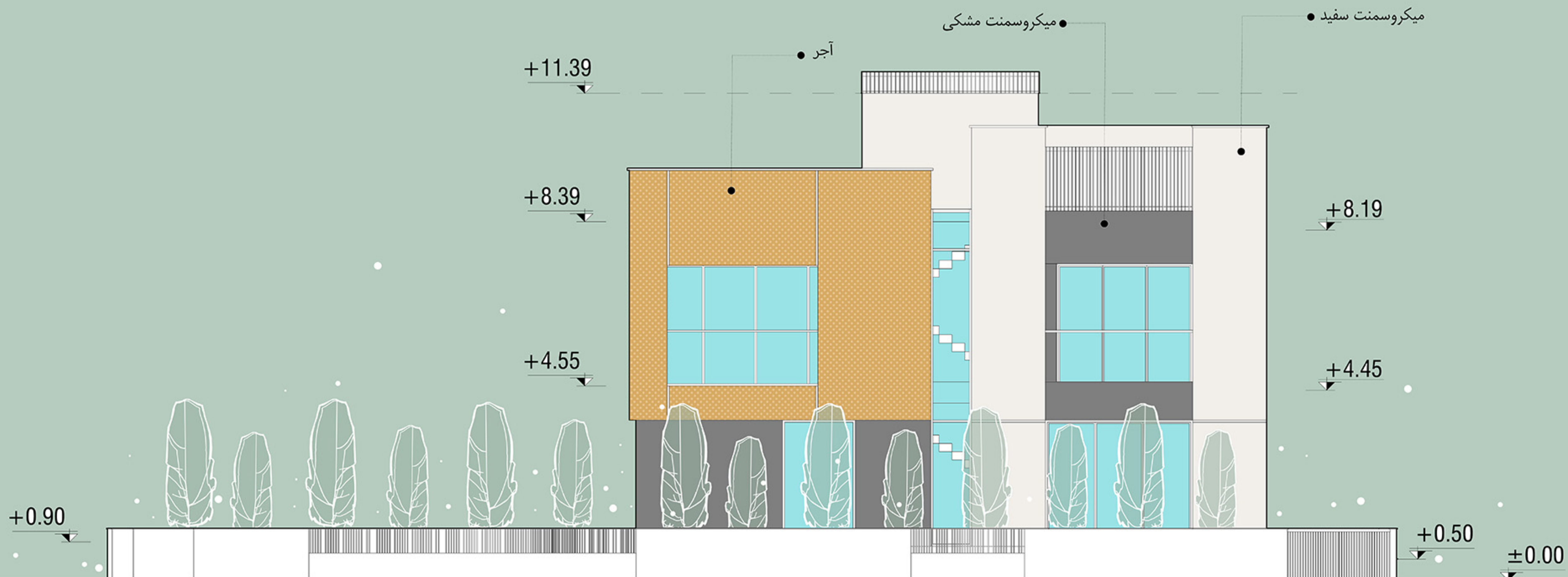
نمای شمالی (رو به کوه های نمک آبرود)
