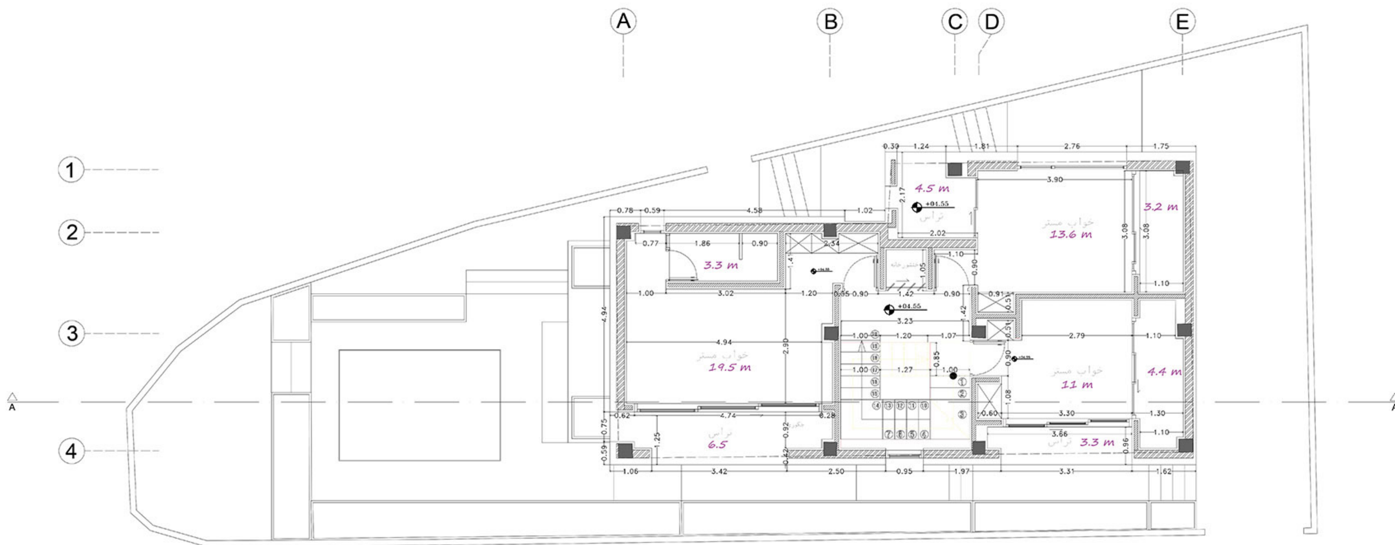
پلان اندازه گذاری طبقه ی همکف در ارتباط با محوطه
