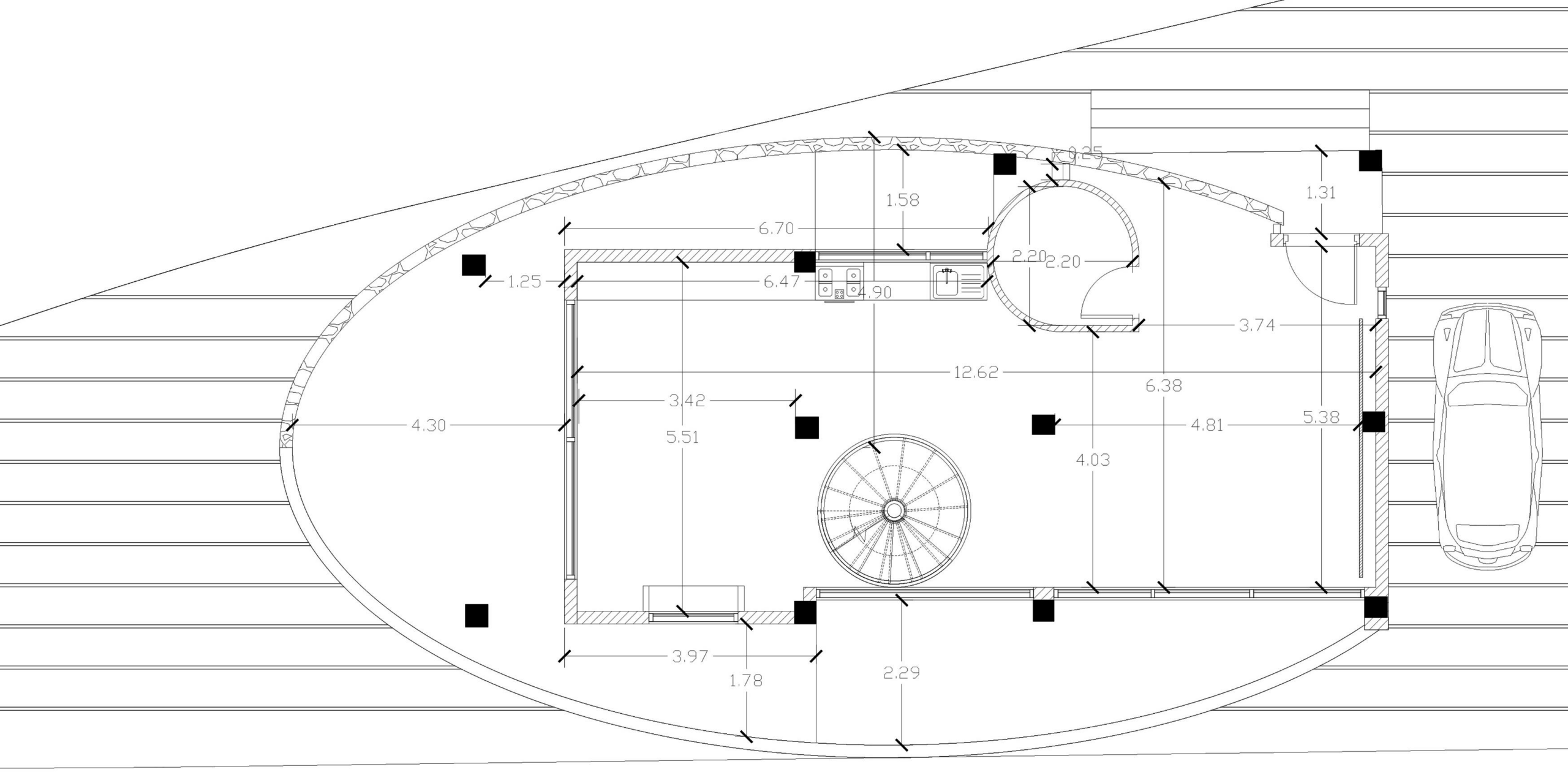
پلان اندازه گذاری طبقه همکف
