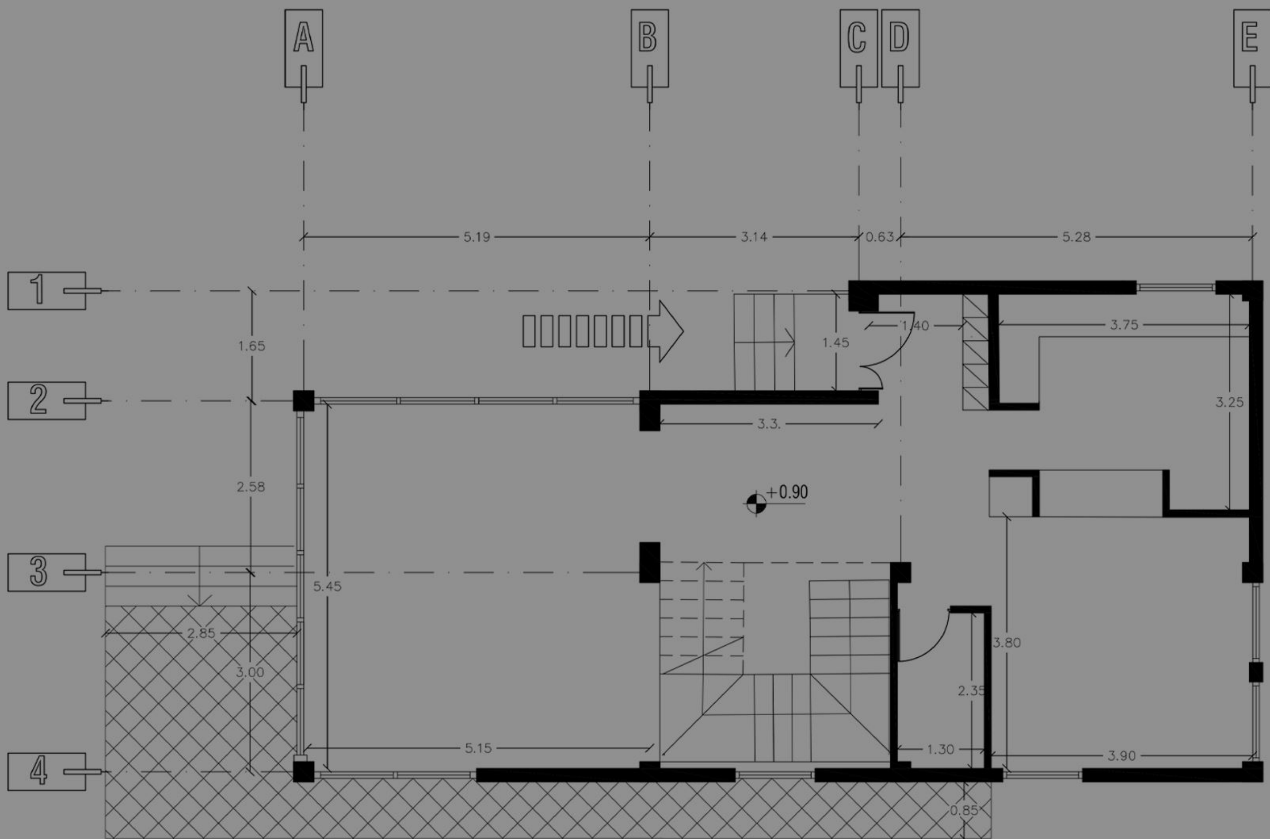
پلان اندازه گذاری همکف
