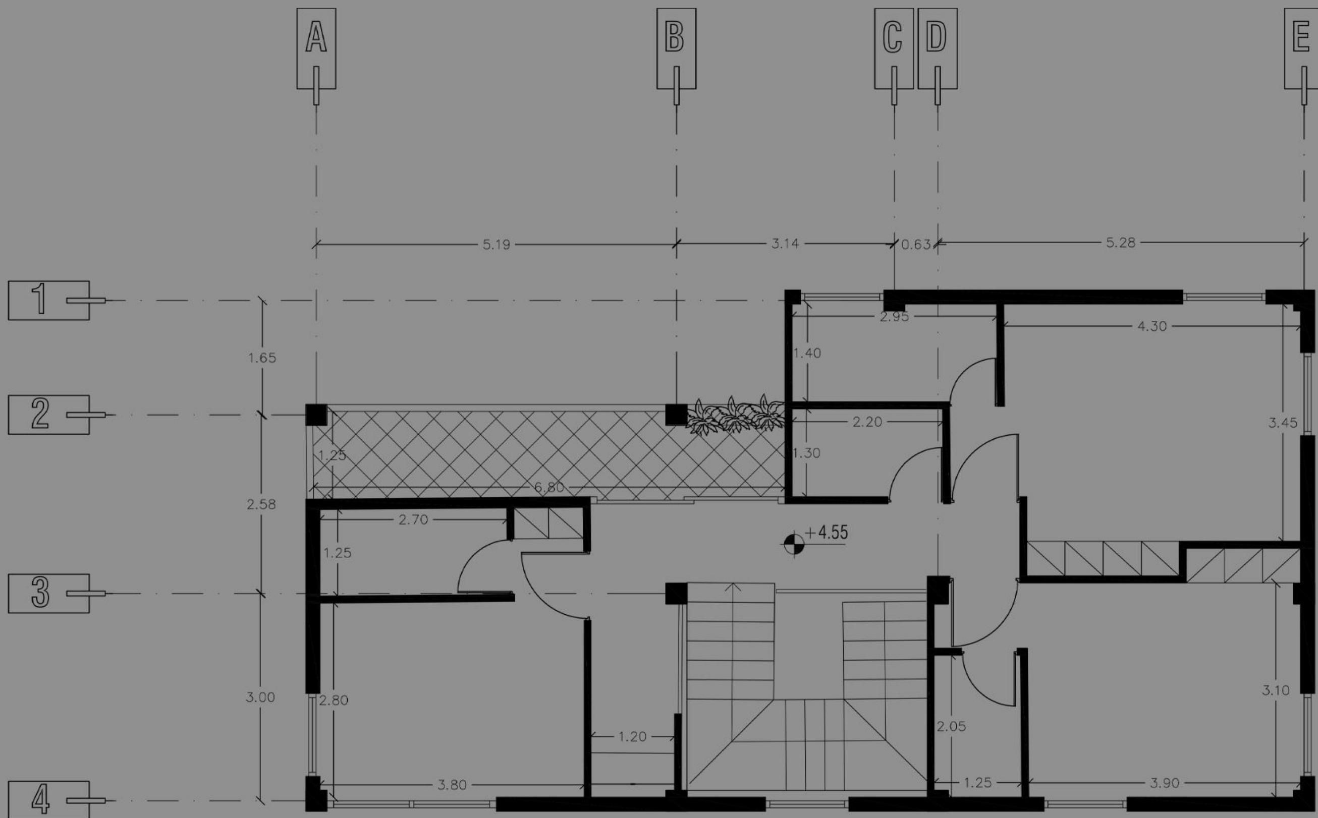
پلان اندازه گذاری طبقه اول
