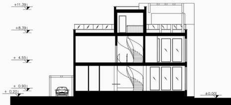
B-B SC . 1:100
