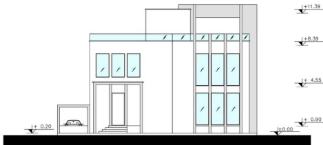
نمای شمالی SC . 1:100
