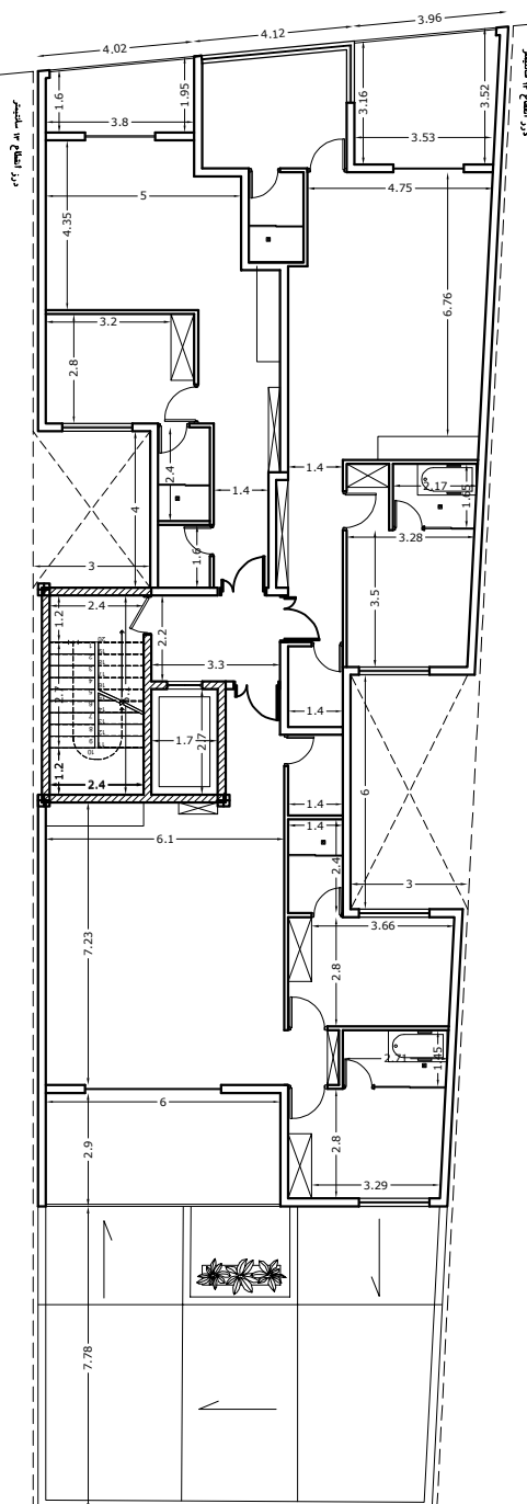
پلان طبقات ۱ و ۳ و ۵
