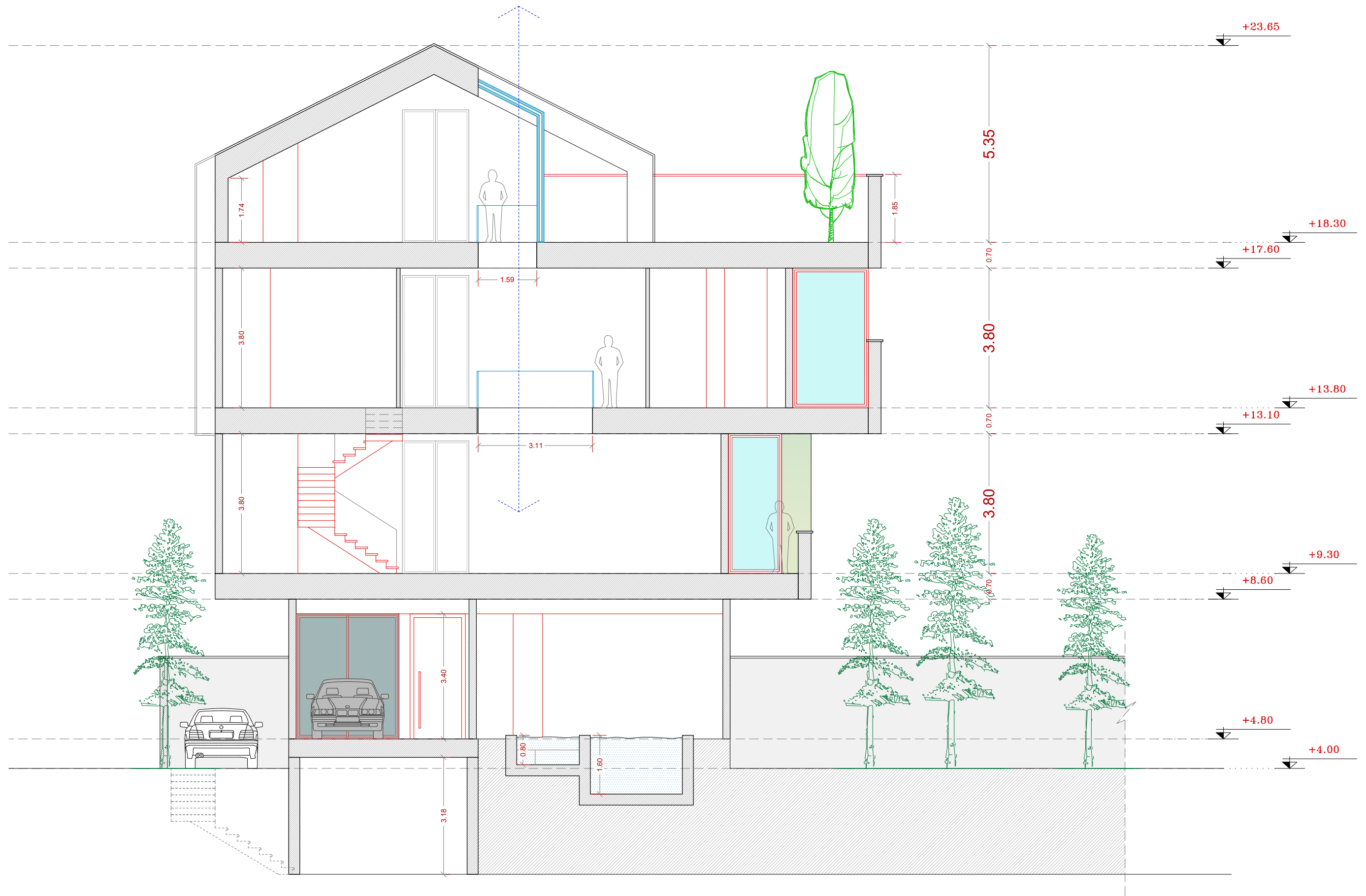
SECTION A-A
