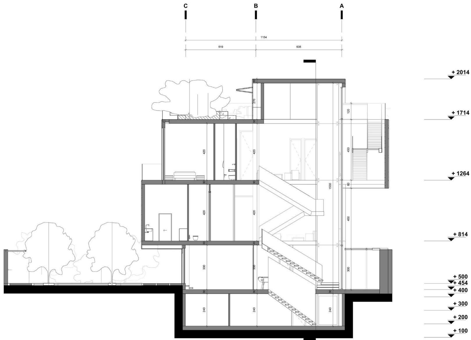
Section A-A
