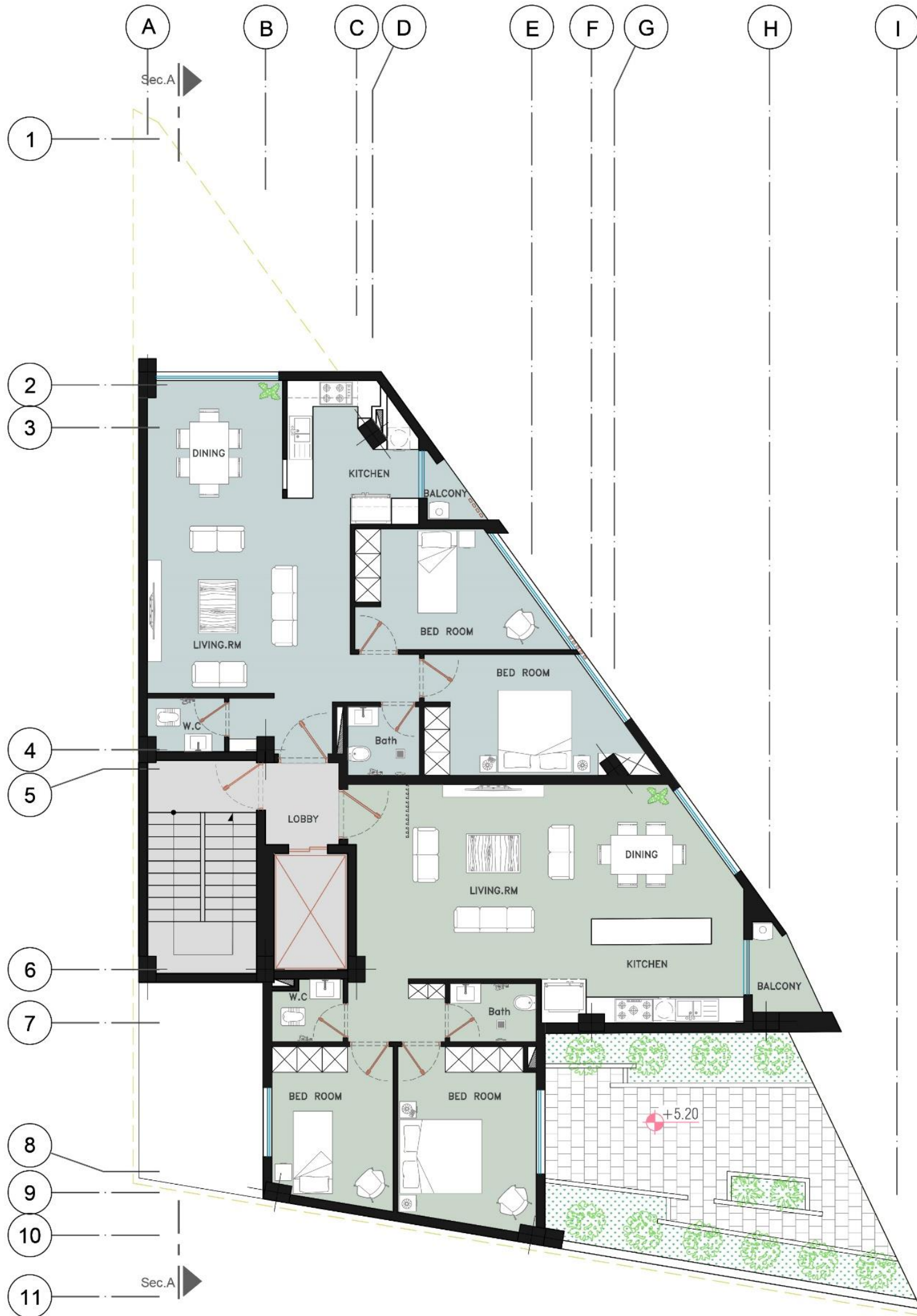
پلان مبلمان طبقات مقیاس: ۱/۱۰۰
