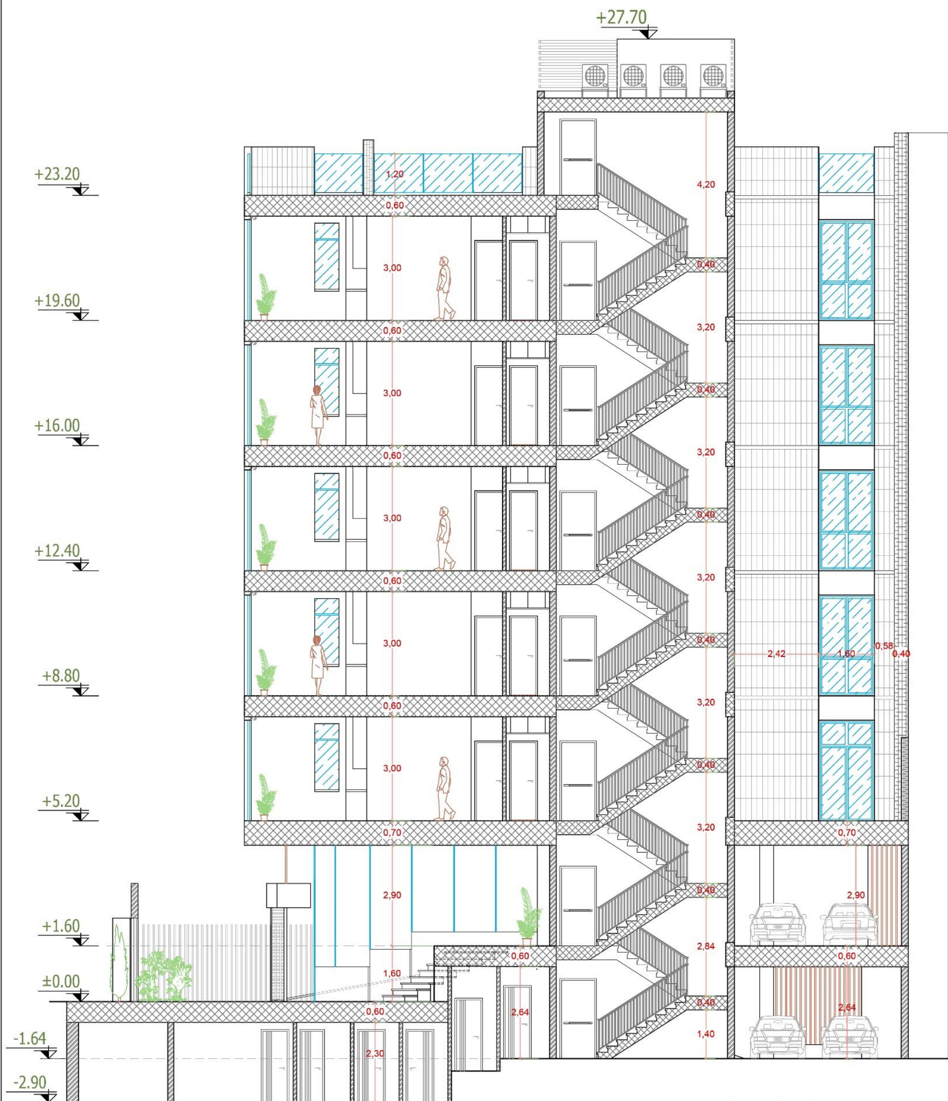
برش A-A مقیاس: ۱/۱۰۰
