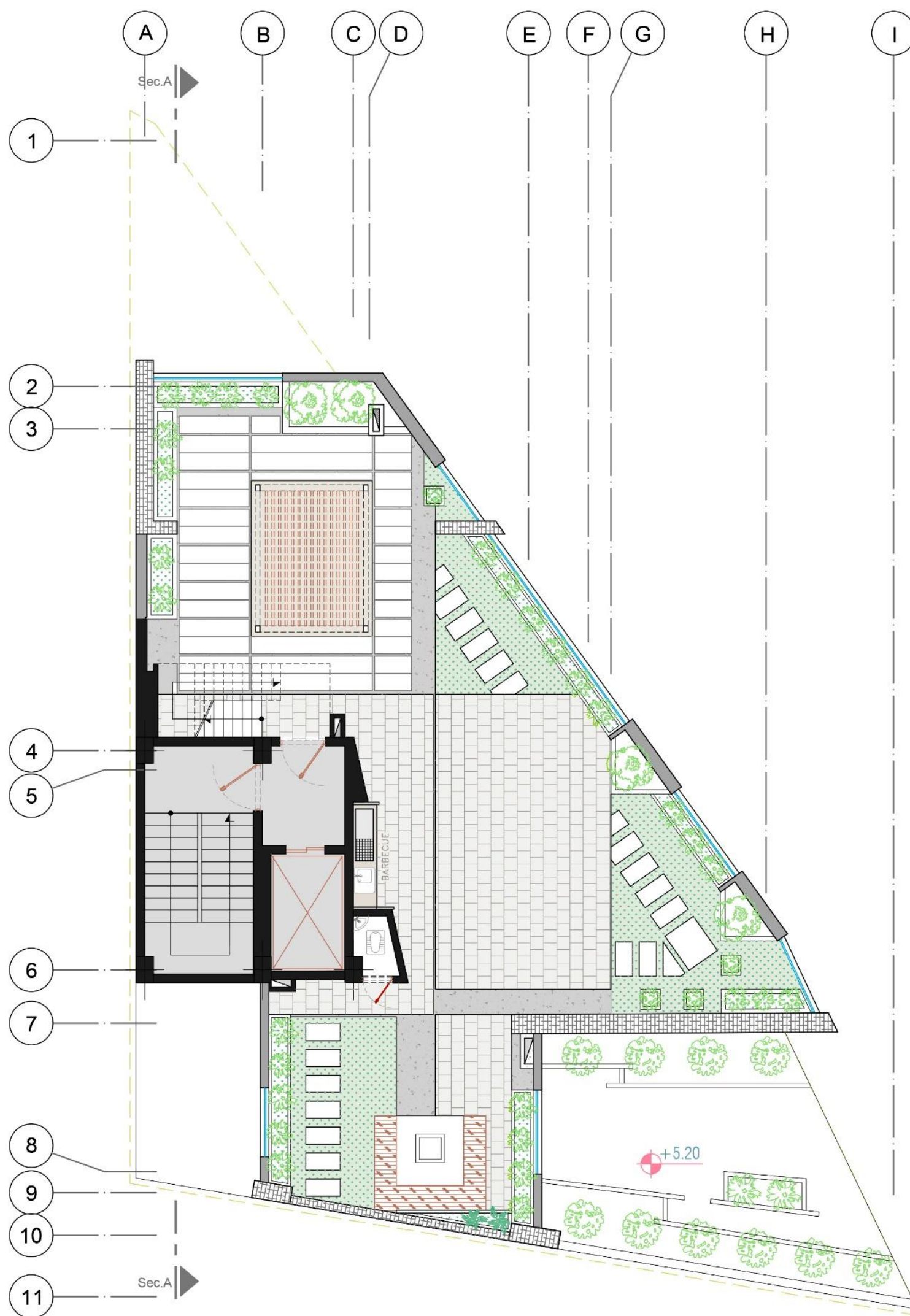
پلان مبلمان روف گاردن مقیاس: ۱/۱۰۰
