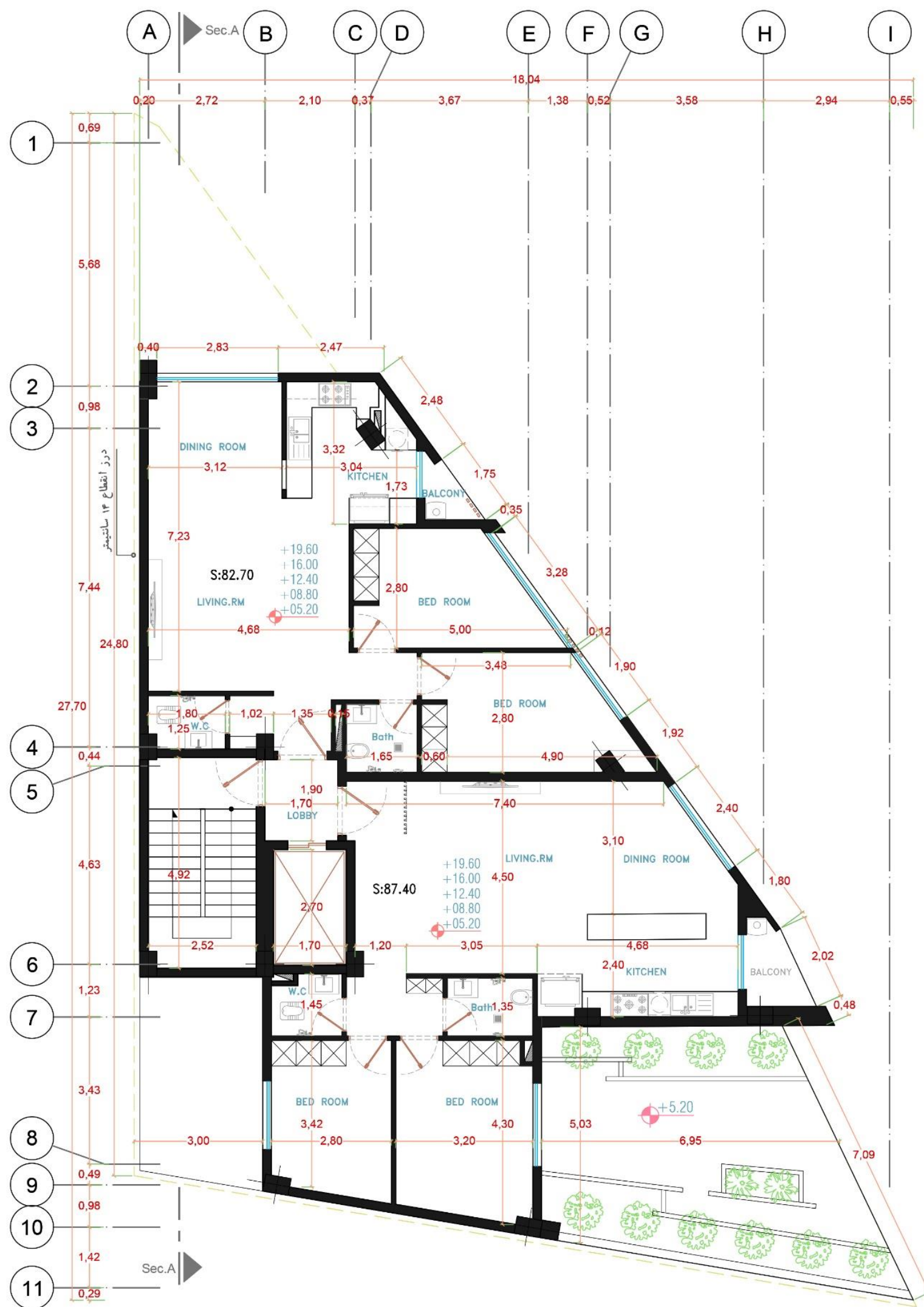
پلان اندازه گذاری تیپ طبقات مقیاس: ۱/۱۰۰
