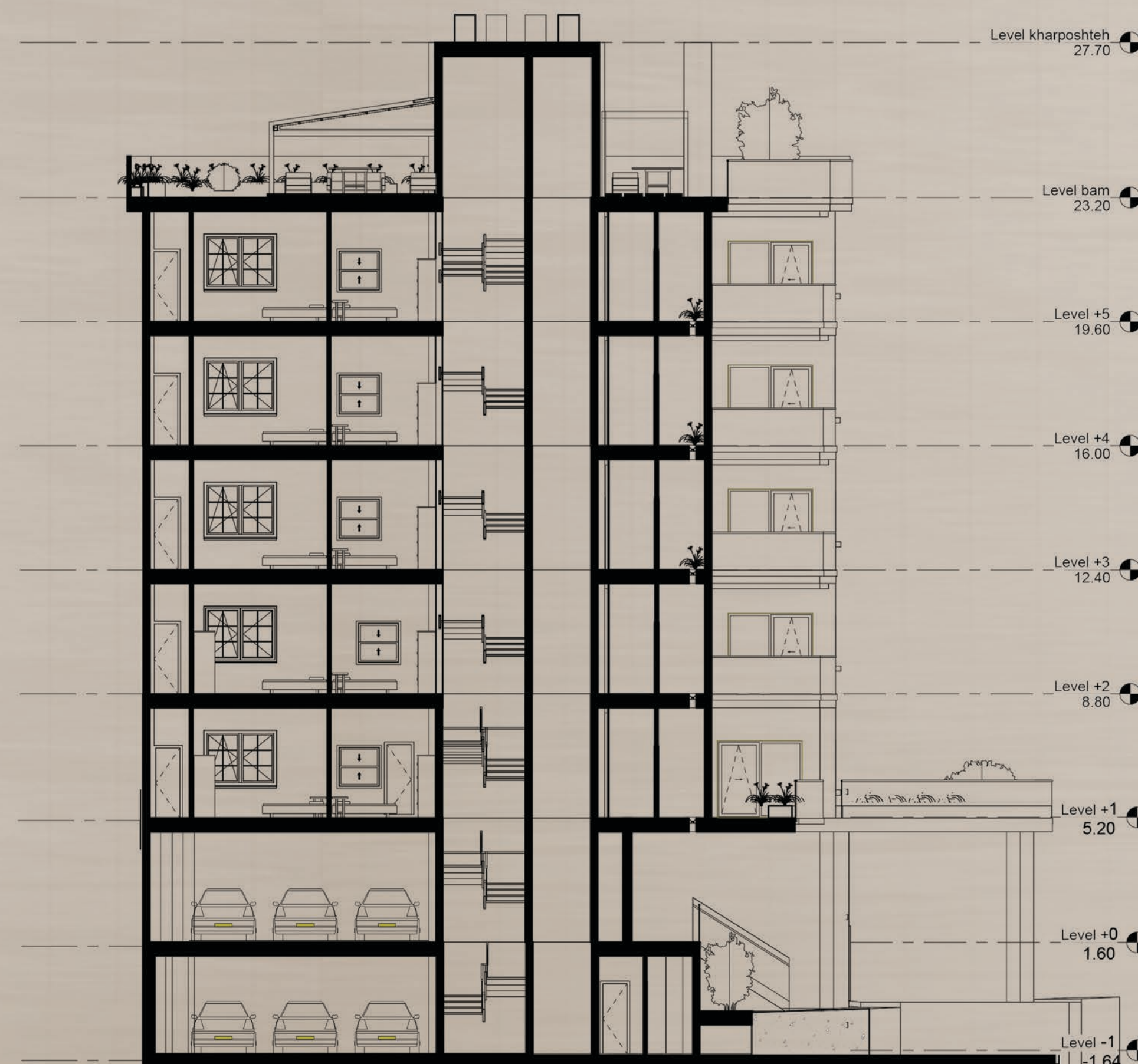
مقطع طولی
