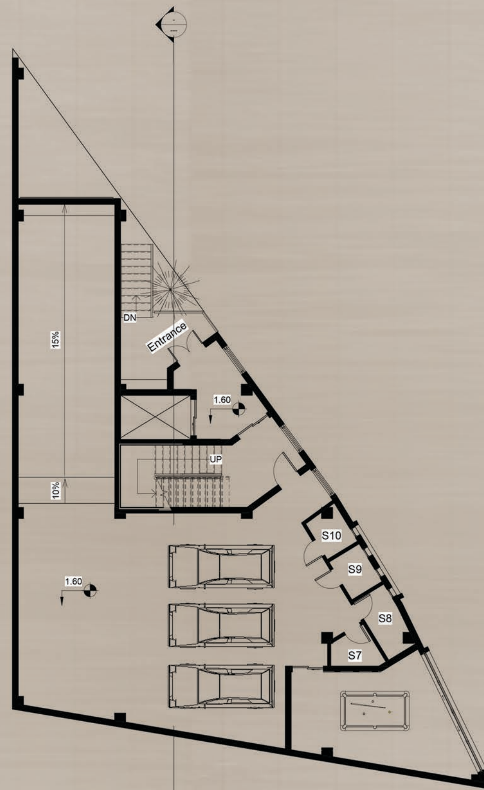
پلان همکف
