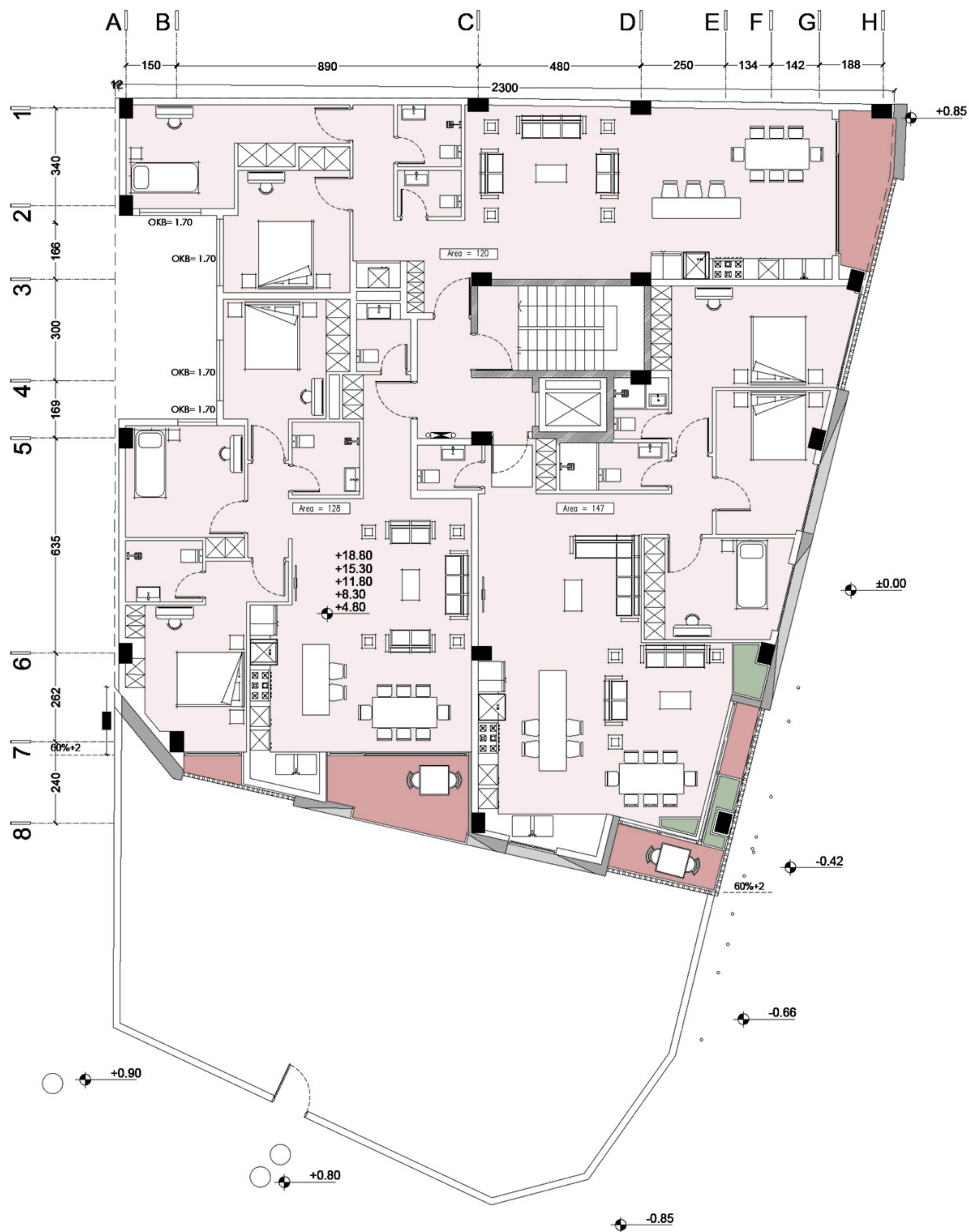
پلان طبقه ی اول (تاثیر نما)
