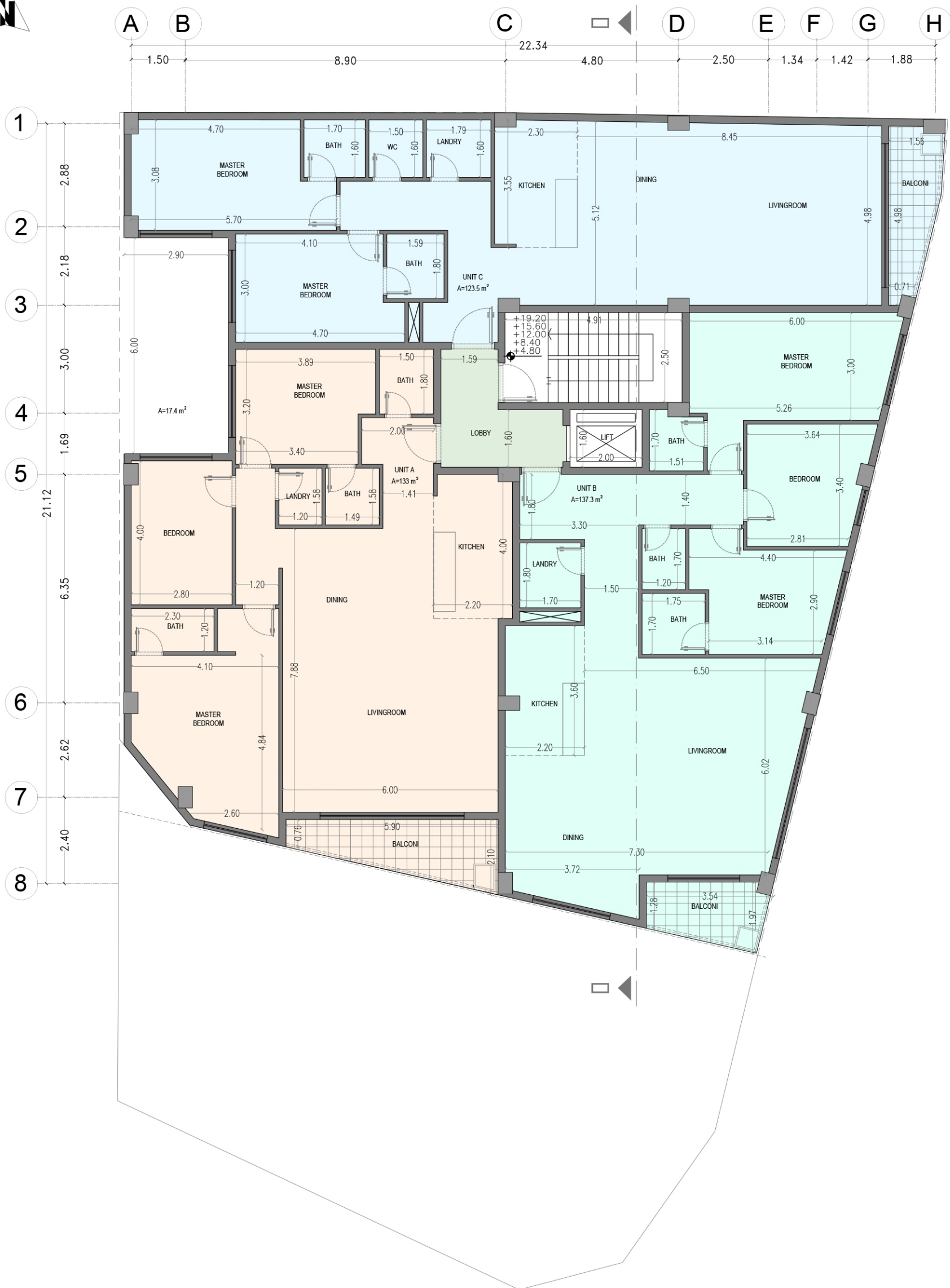
پلان اندازه گذاری طبقات (طبقه اول تا پنجم)
