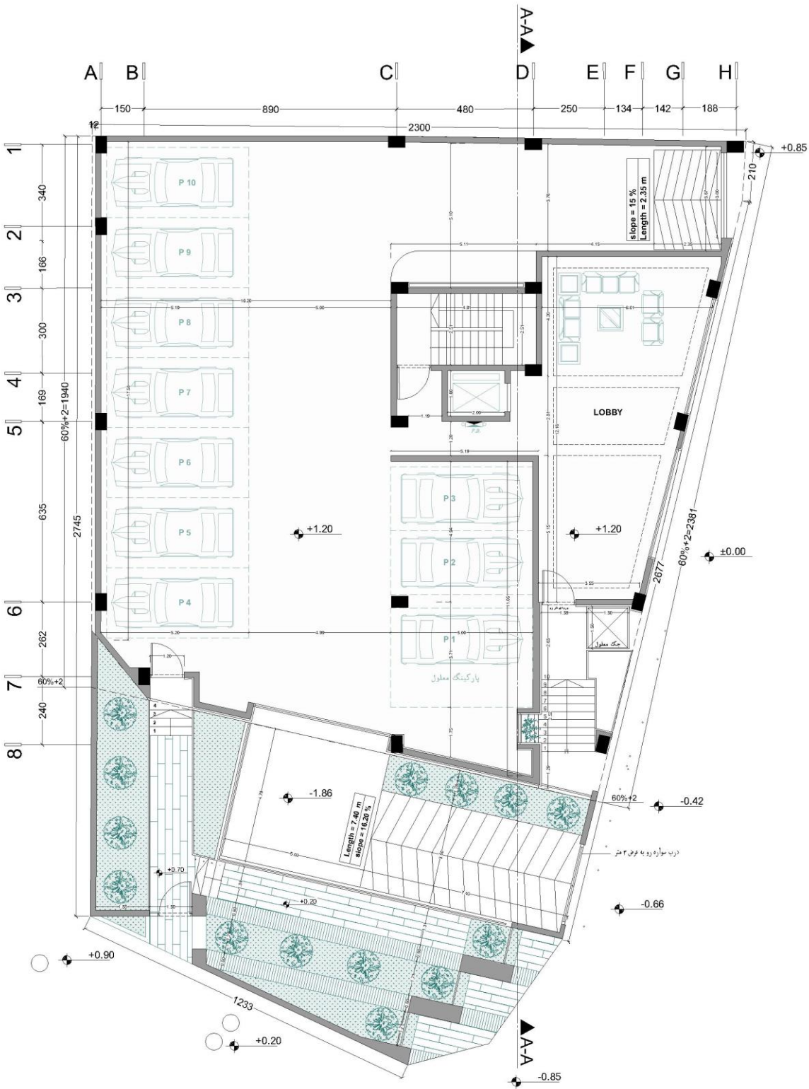
پلان اندازه گزاری طبقه همکف
