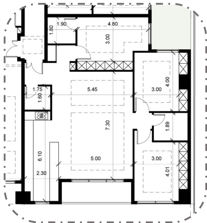
پلان اندازه گذاری
