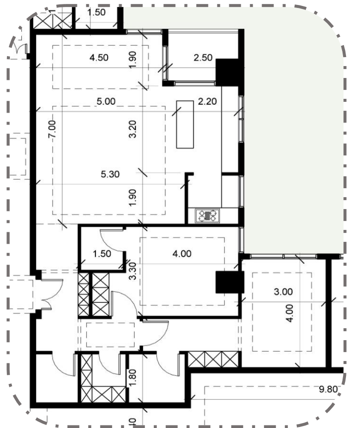
پلان اندازه گذاری
