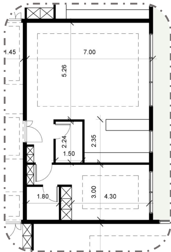
پلان اندازه گذاری
