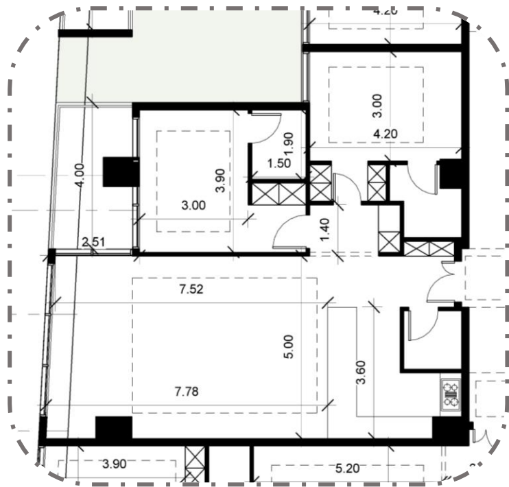
پلان اندازه گذاری
