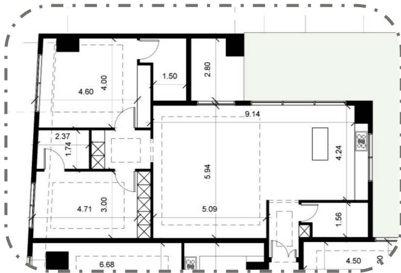
پلان اندازه گذاری
