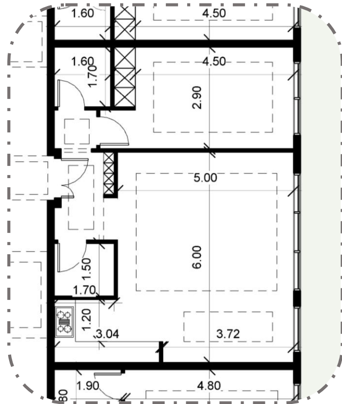
پلان اندازه گذاری
