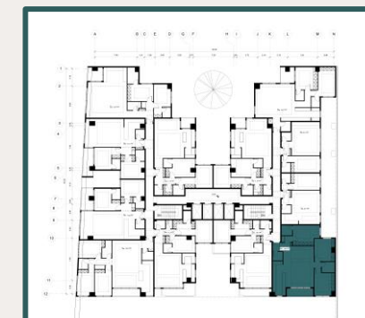
پلان راهنما
