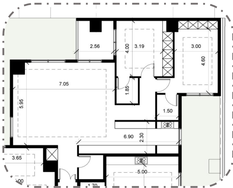
پلان اندازه گذاری
