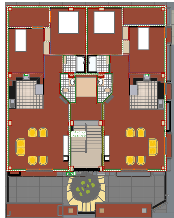
5 eleman6 Axonometry 1:200
